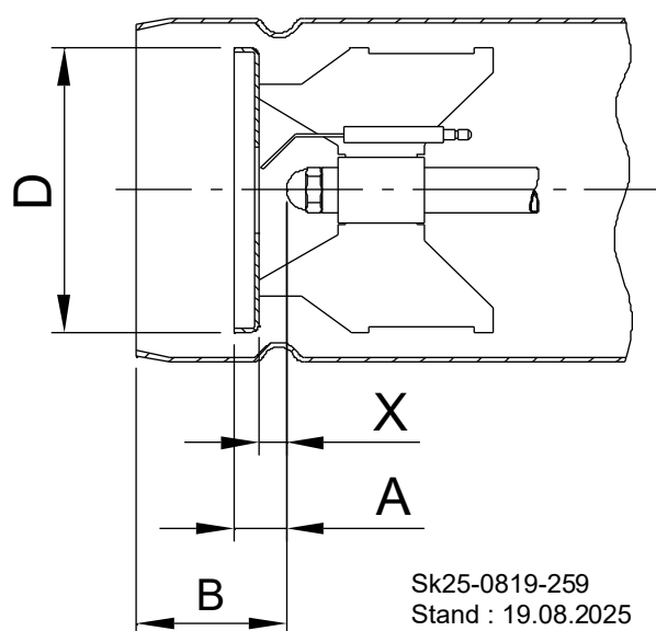
Abb. 29: Einstellmaße SL 400/2
