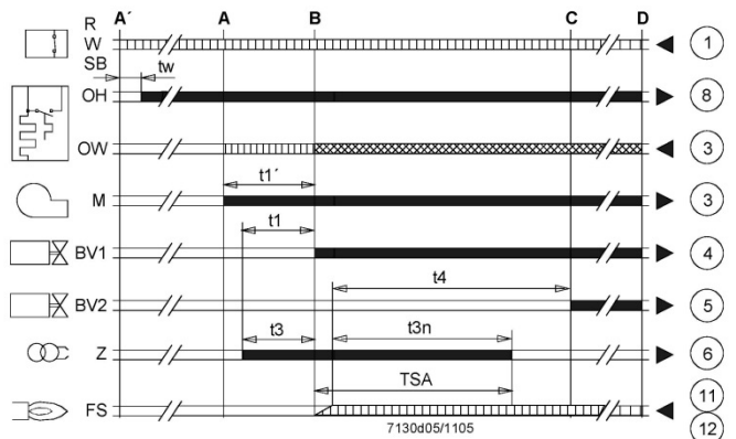
Abb. 18: Programmablauf LMO 44.255
