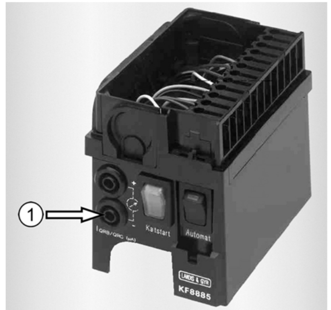
Abb. 22: Prüfsockel KF 8885 (auf Anfrage) Messanschluss Flammenüberwachung ①
