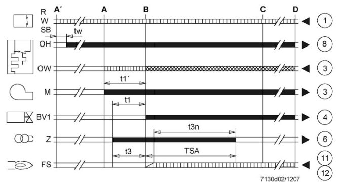
Abb. 16: Programmablauf LMO 14
