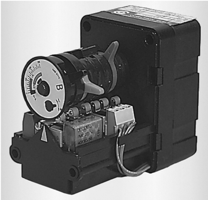
Abb. 14: Stellmotor LKS 130
