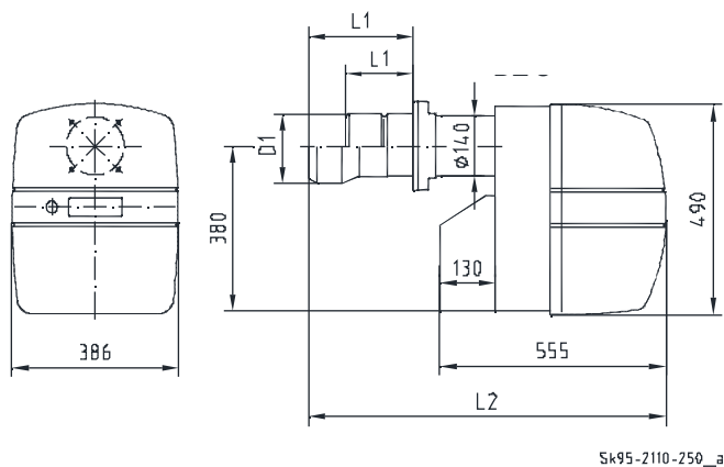
Abb. 2: Brennerabmessungen SL 400/2 – SL 420/2
