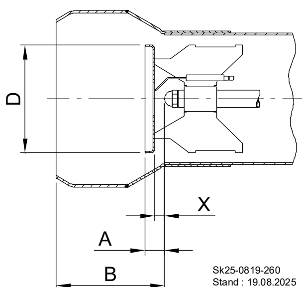
Einstellmaße SL 410 – SL 420/2
