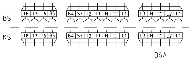
Abb. 4: Elektroanschluss
