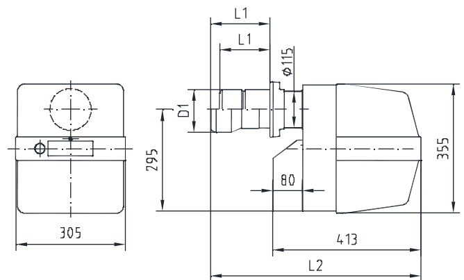
Abb. 1: Brennerabmessungen SL 44 – SL 66/2
