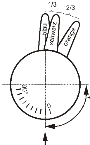
Abb. 12: Schaltpunkt Magnetventil
