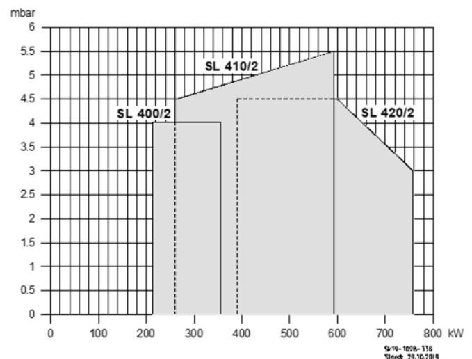
Abb. 28: Leistungsdiagramm SL 400/2 – SL 420/2
