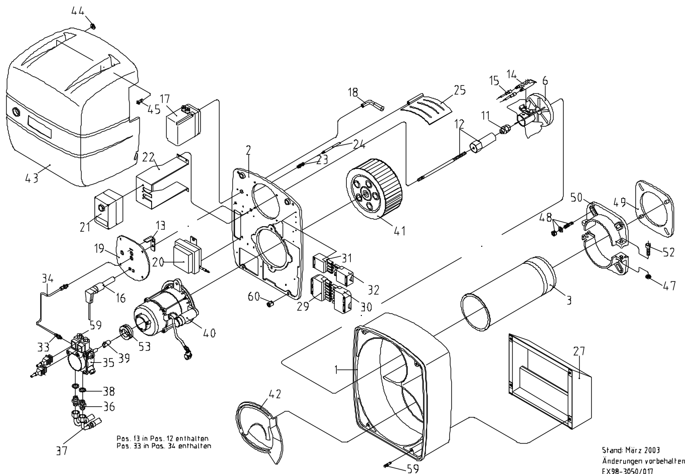
Abb. 24: Explosionszeichnung SL 400/2
