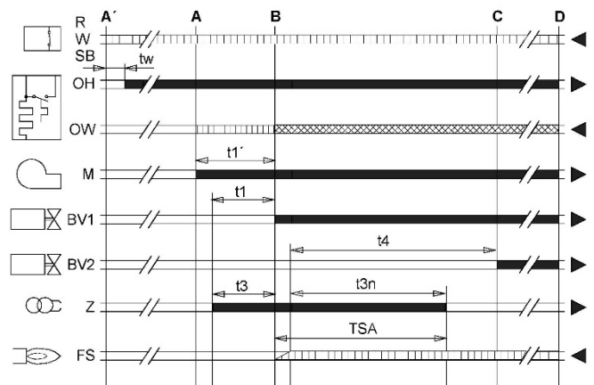
Abb. 17: Programmablauf LMO 24
