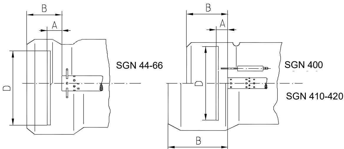
Abb. 32: Einstellmaße
