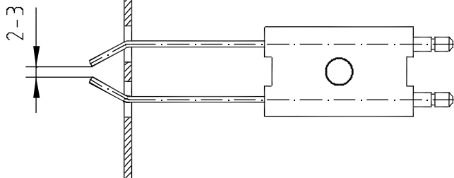
Abb. 23: ZündelektrodenEinstellung Erdgas und Flüssig- gas [SGN(F) 44-420/2]
