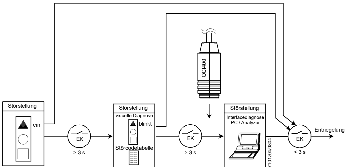
Abb. 30: Ablauf Störursachendiagnose EK = Entstörtaster
