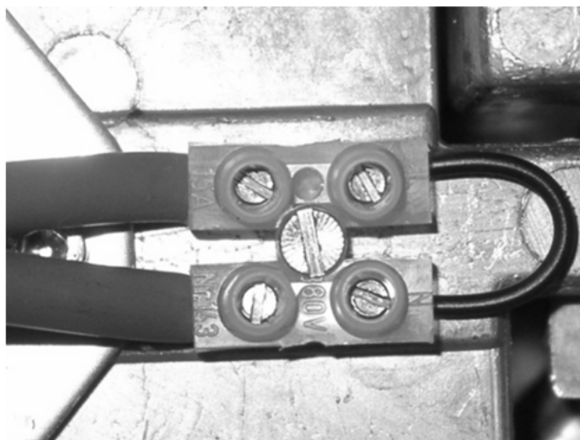
Abb. 26: Lusterklemme zur Messung des Ionisationsstromes
