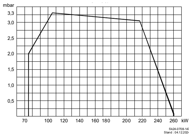
Abb. 34: Arbeitsfeld der Gasbrenner SGN(F) 55/2
