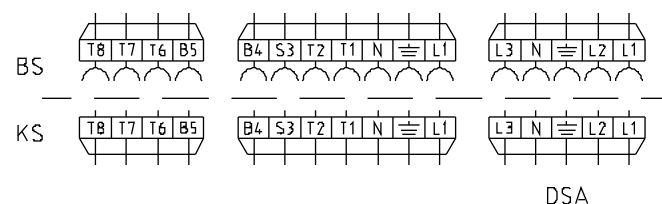
Abb. 11: Elektroanschluss
