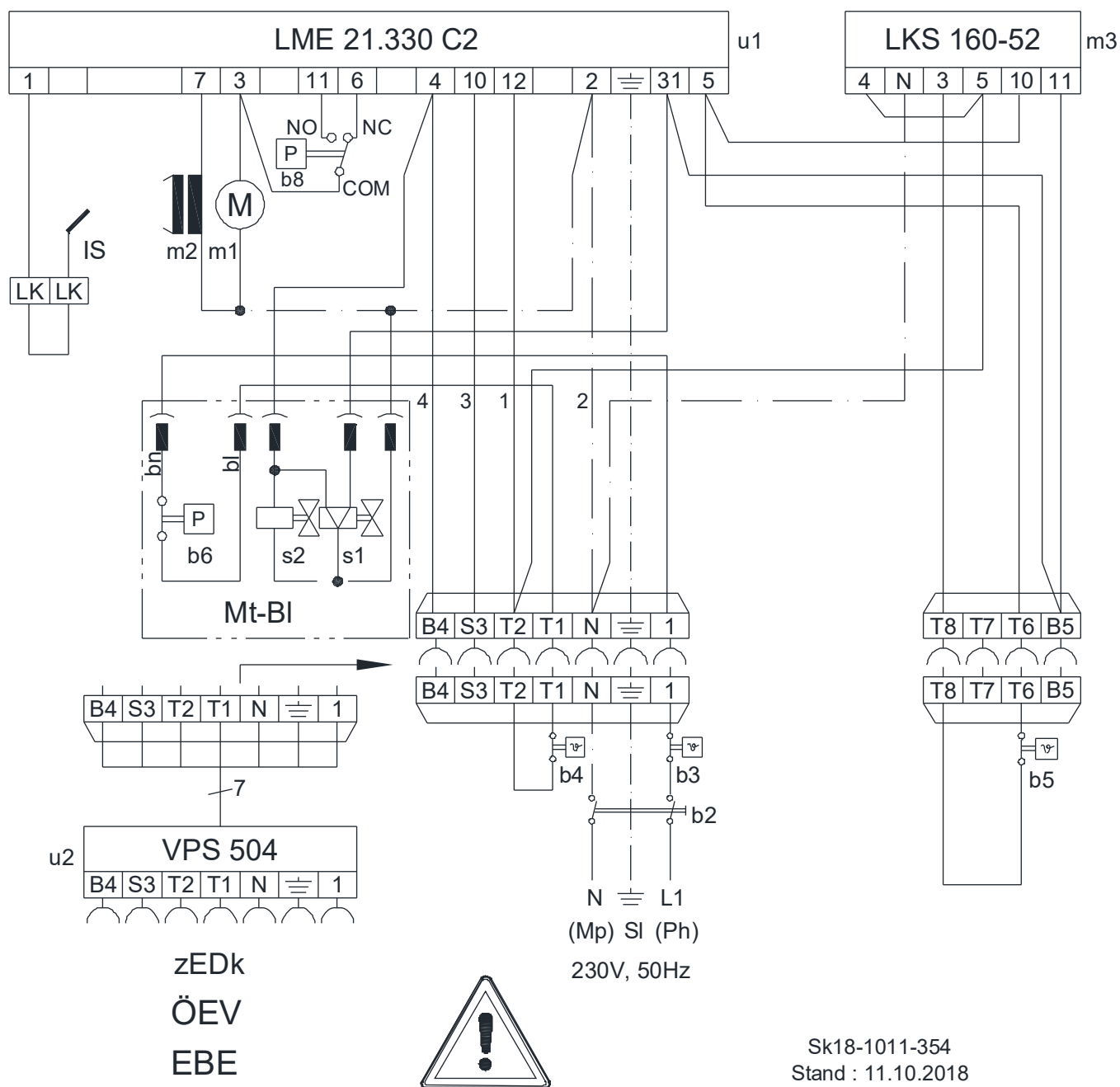
Abb. 14: Schaltplan SGN(F) 400/2 (zweistufig) mit Siemens LME 21 und LKS 160
