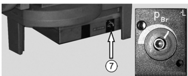
Abb. 16: Gasdruckverstellung ⑦
