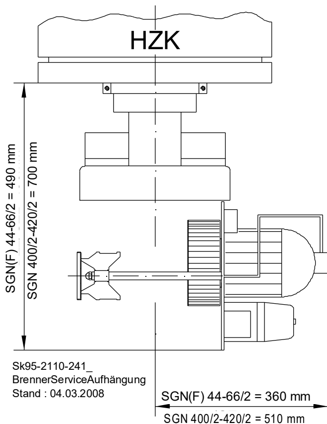
Abb. 22: Brenner in Service-Aufhängung
