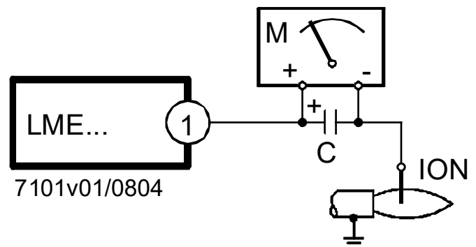
Abb. 25: Mess-Schaltung LME 21
