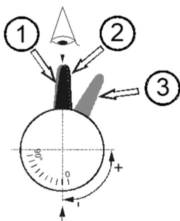
Abb. 6: Luftklappenantrieb Stufe 1
