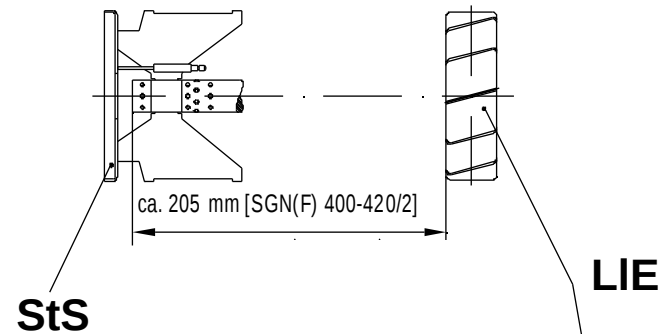
Abb. 19: Position Luftleiteinrichtung SGN(F) 400/2-420/2
