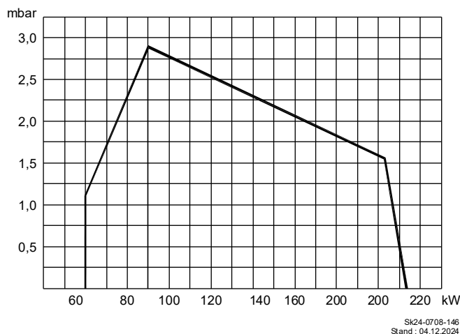
Abb. 33: Arbeitsfeld der Gasbrenner SGN(F) 44/2
