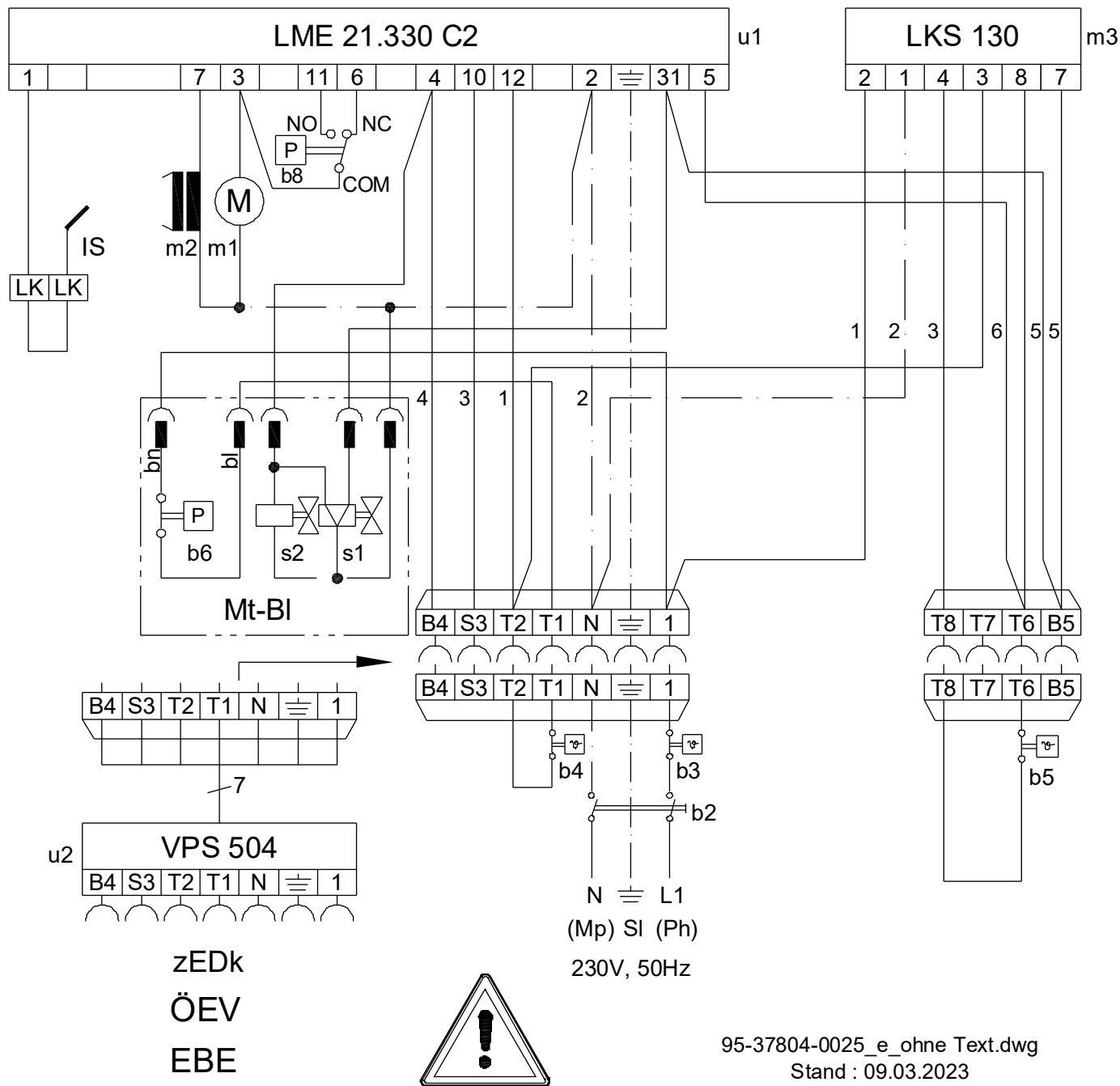
Abb. 13: Schaltplan SGN(F) 44/2-66/2 (zweistufig) mit Siemens LME 21 und LKS 130
