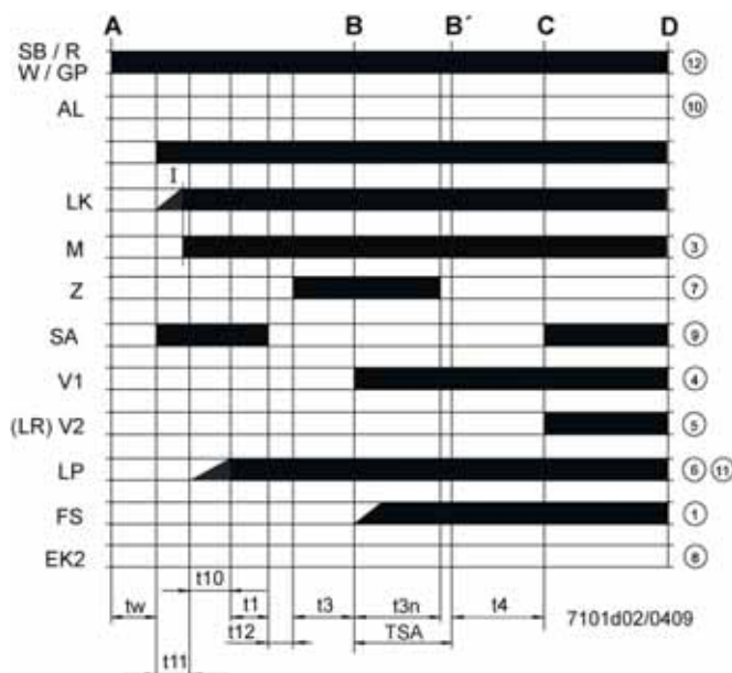
Abb. 21: Programmablauf LME 22
