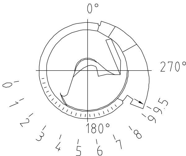
Abb. 18: Verstellen der Lufteinlaufdüse beim SGN(F) 44-420/2
