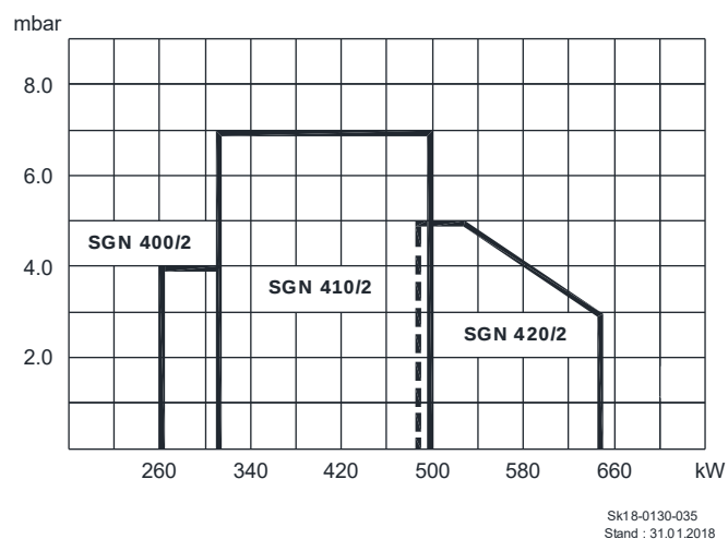
Abb. 36: Arbeitsfeld der Gasbrenner SGN(F) 400/2-420/2
