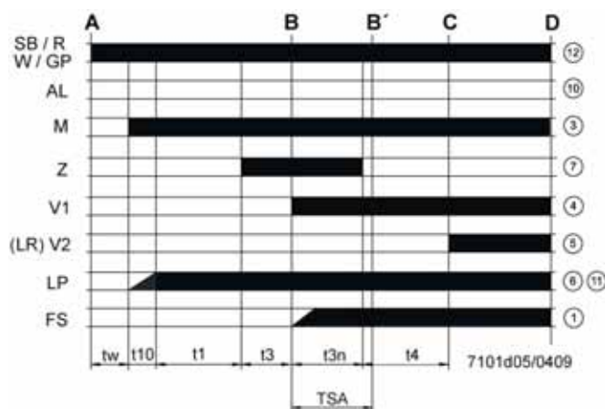
Abb. 20: Programmablauf LME 21
