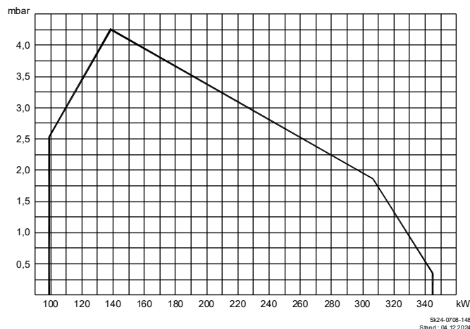
Abb. 35: Arbeitsfeld der Gasbrenner SGN(F) 66/2
