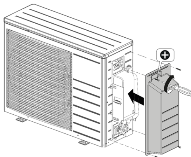
Abb. 26: Montage der Seitenverkleidung
