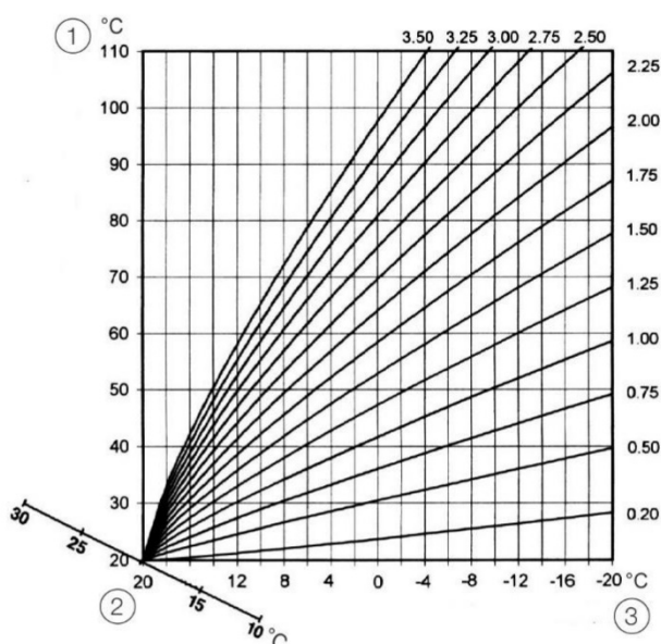
Abb. 7: Heizkurve
