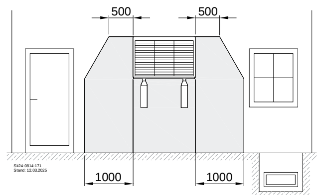
Abb. 4: Schutzbereich Wandmontage
