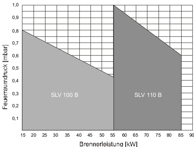
Abb. 20: Leistungsdiagramm
