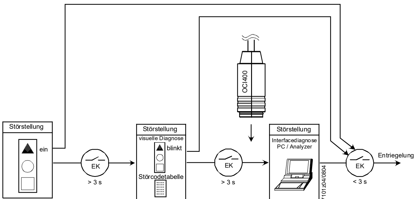
Abb. 23: Ablauf Störsachendiagnose EK = Entstörtaster
