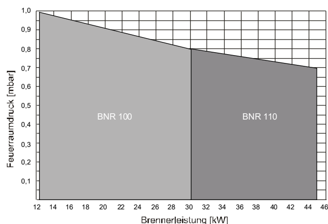
Abb. 25: Leistungsdiagramm
