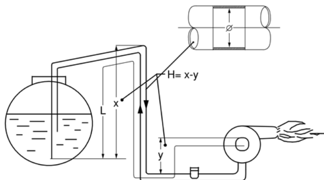
Abb. 7: Zweistranganlagen mit höher liegendem Tank
