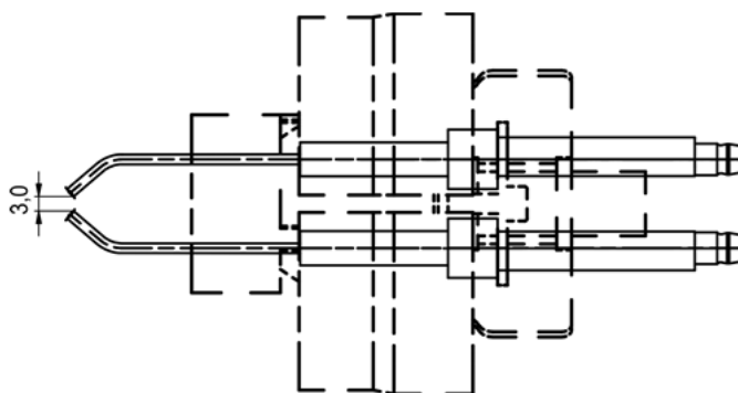
Abb. 21: Zündelektrodeneinstellung
