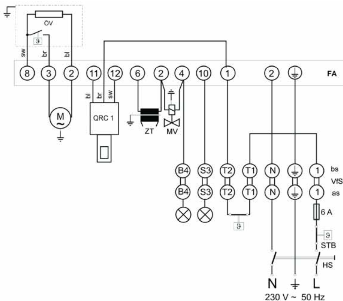
Abb. 9: Schaltplan für Feuerungsautomat Siemens
