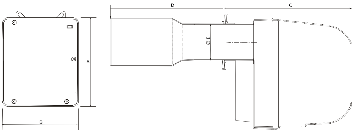
Abb. 1: Abmessungen
