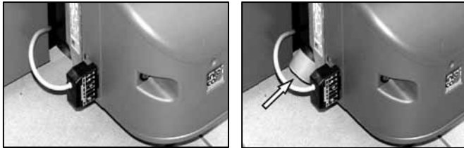
Abb. 16: Brenner ohne und mit Luftstutzen
