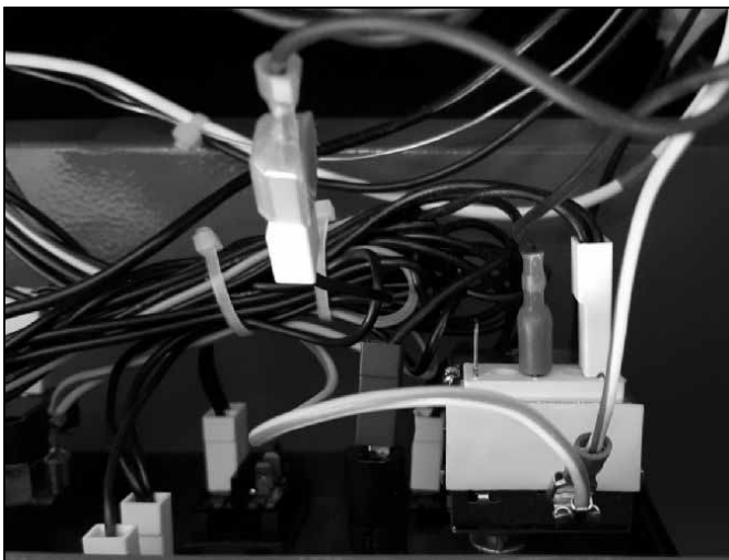
Abb. 38: Reihenschaltung der Sicherheitsthermostaten und Kombination der Schutzleiteranschlusstecker.
