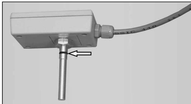
Abb. 90: Dichtung am Temperaturfühler des ATB DN80
