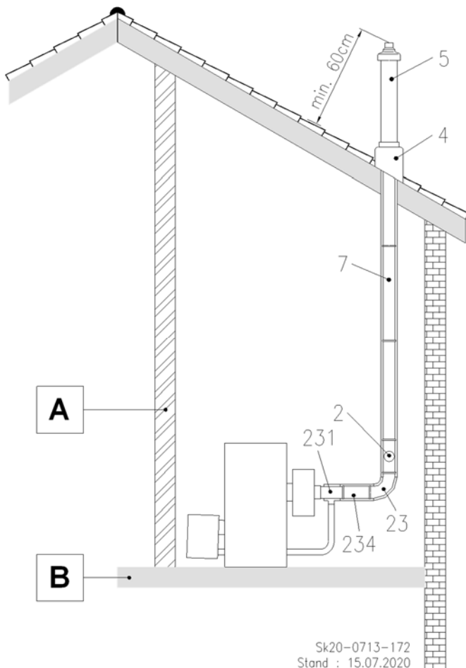
Abb. 49: C 33x Dachheizzentrale mit der Durchführung senkrecht durch ein Schrägdach
