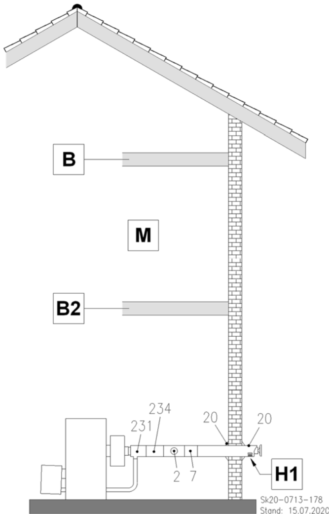
Abb. 47: C 13x Luft-Abgas-Rohrsystem horizontal durch die Außenwand
