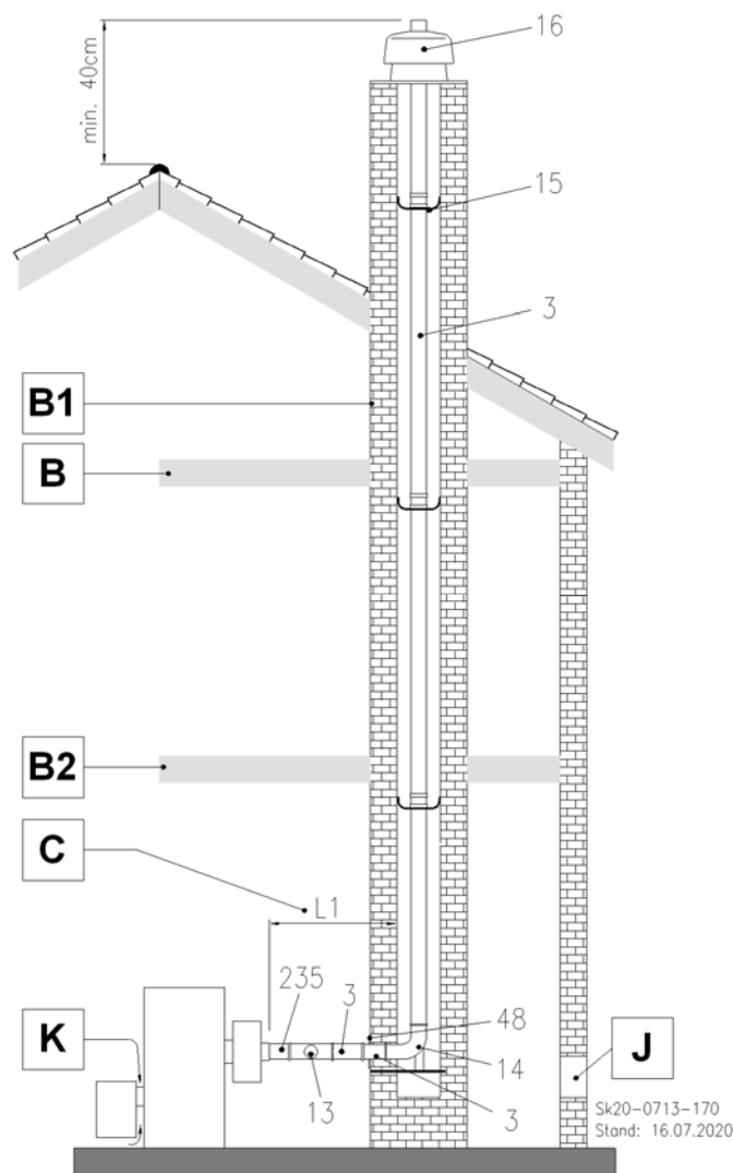
Abb. 45: B 23 Abgasrohr im Schornsteinschacht
