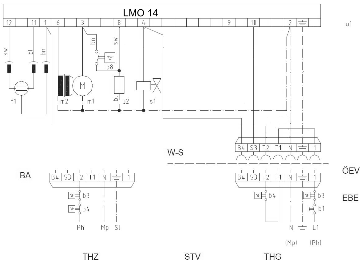
Abb. 42: Schaltplan Blaubrenner BNR 100 mit Siemens Feuerungsautomat LMO 14
