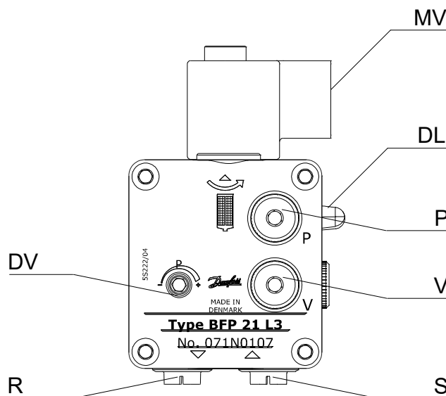
Abb. 78: Danfoss Ölpumpe BFP 21 L3 (Druckbereich 10-14 bar)
