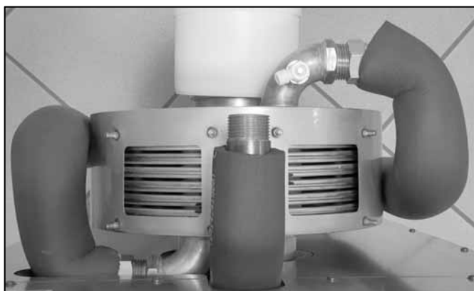
Abb. 82: Reinigungsöffnungen des Abgaswärmetauschers
