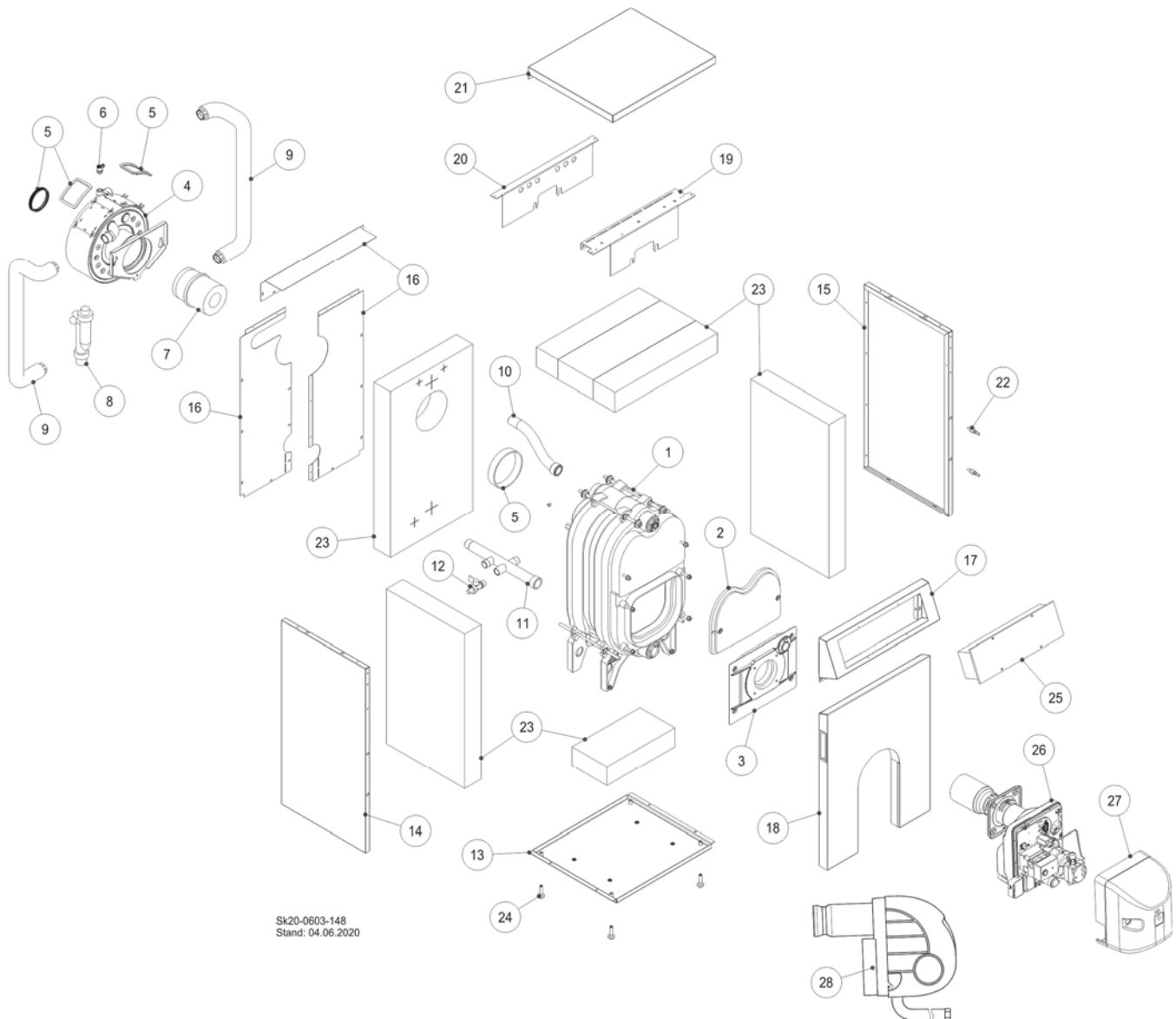
Abb. 94: Explosionsdarstellung RATIOLINE Plus
