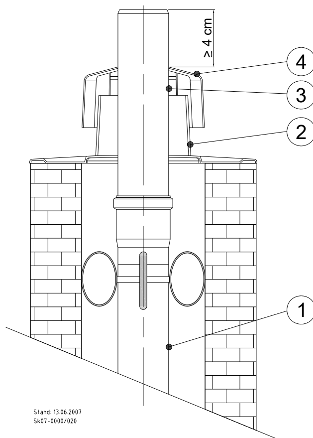
Abb. 59: Schachtabdeckung
