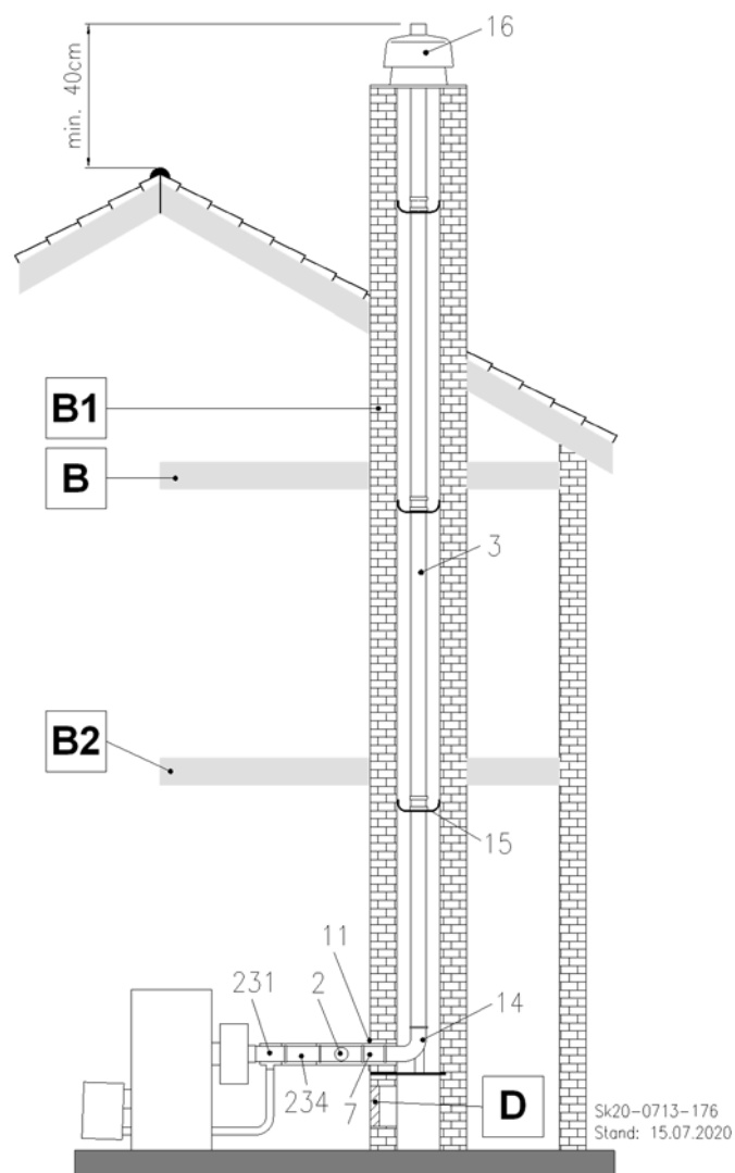
Abb. 54: C 93x Abgasrohr im Schacht
