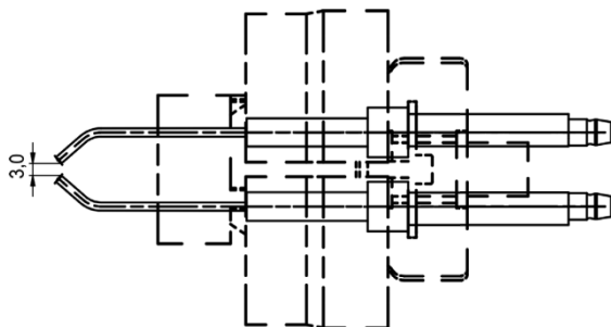
Abb. 93: Der Elektrodenabstand ist 3,0 mm
