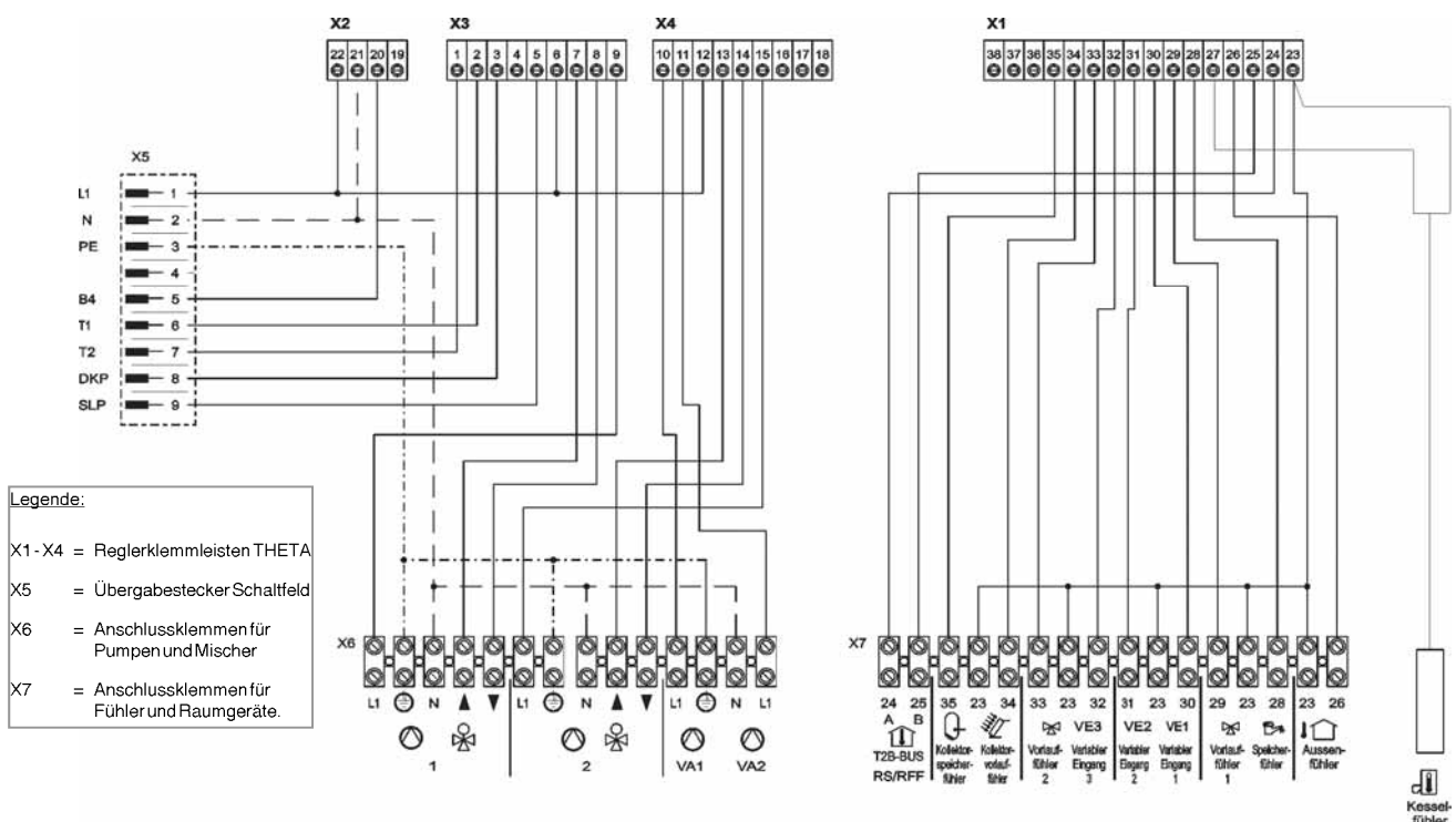
Abb. 41: Schaltplan Regleranschlusskabelbaum THETA+ 233B THETA+ 2233 BVVC-OT
