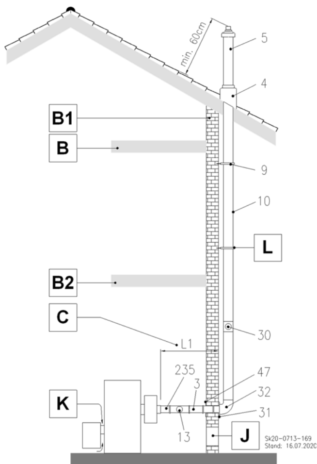
Abb. 44: B 23 Abgasrohr an der Außenwand
