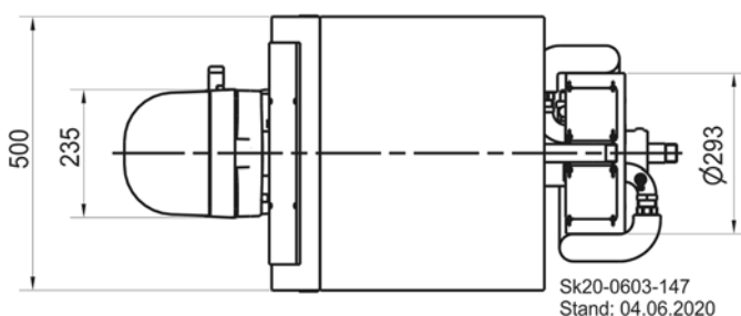
Abb. 3: Abmessungen
