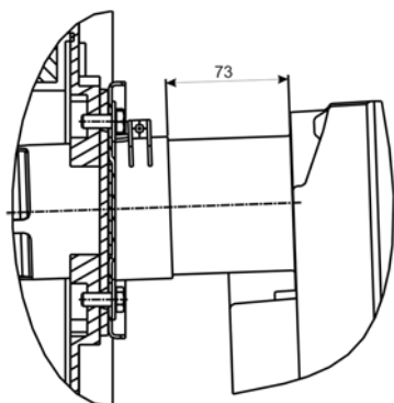
Abb. 72: Brenner-Einschubtiefe
