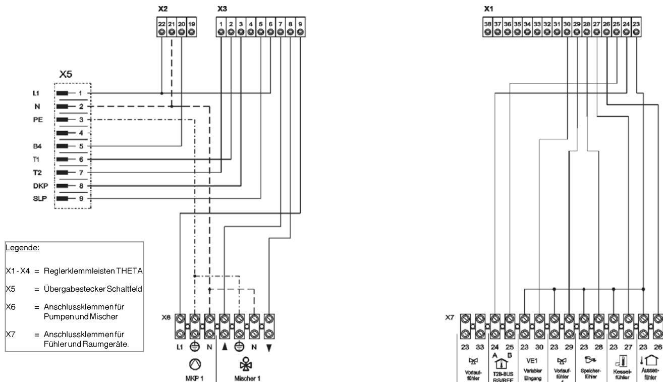
Abb. 40: Schaltplan Regleranschlusskabelbaum für THETA+ 2B und THETA+ 23B
