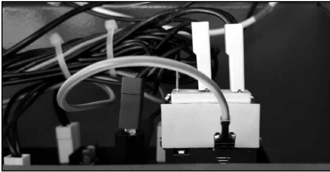
Abb. 36: Aufsicht Kessel-Sicherheitstemperaturbegrenzer (STB) (rechts oben im Kesselschaltfeld)
