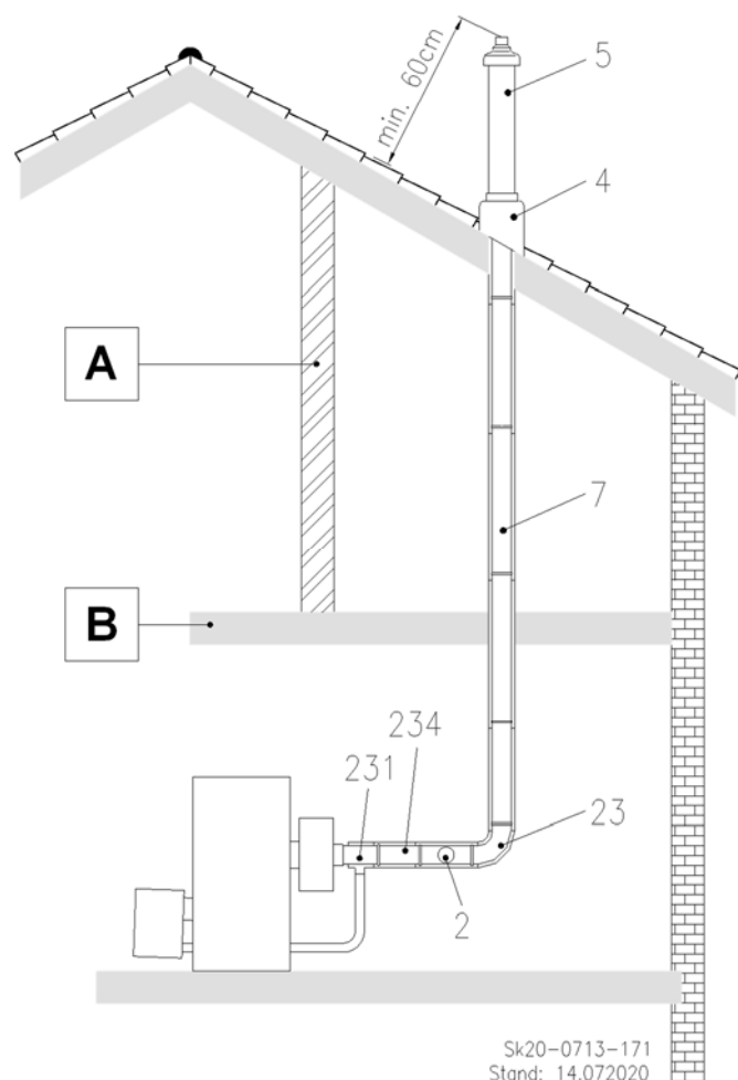
Abb. 48: C 33x Luft-Abgas-Rohrsystem senkrecht durch eine Decke und eine Dachhaut
