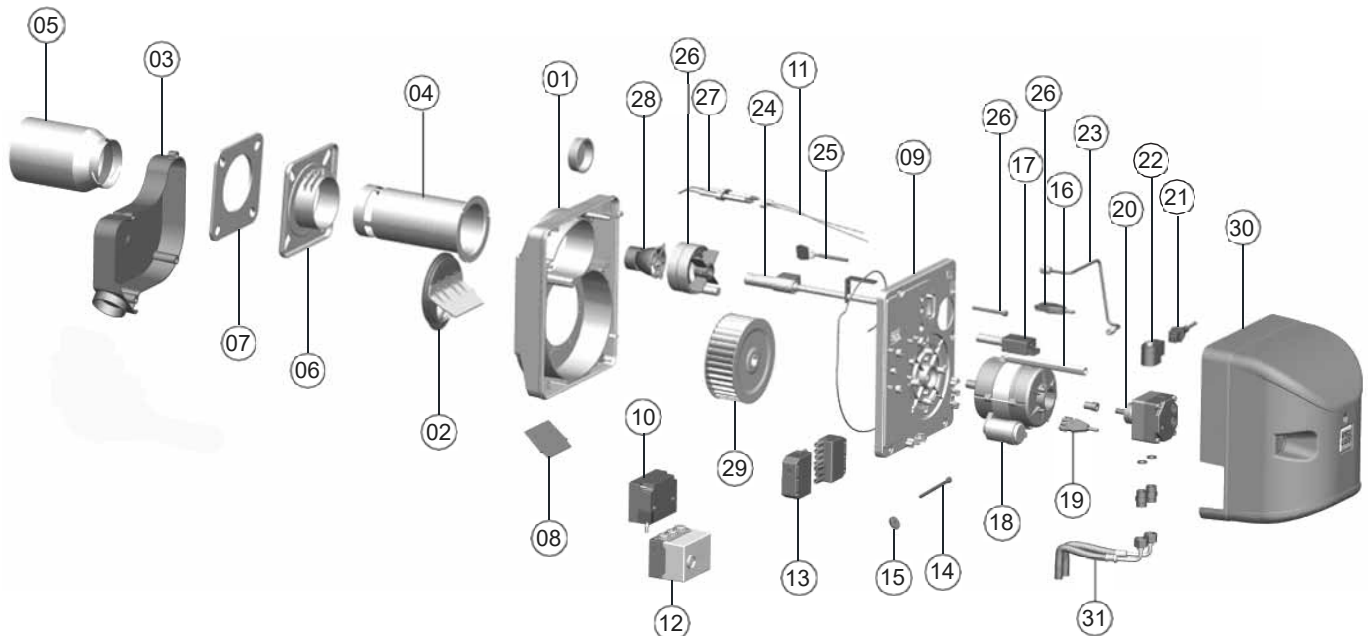
Abb. 95: Explosionsdarstellung Ölbrenner BNR 100
