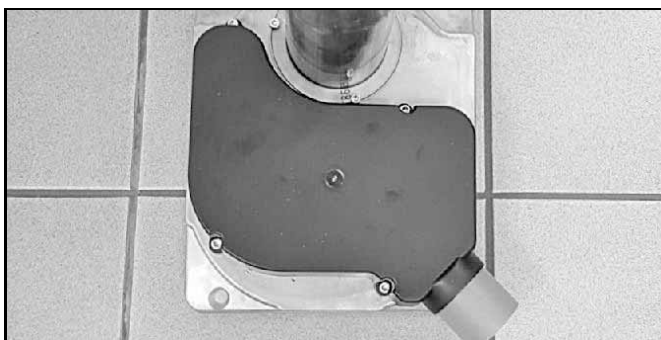
Abb. 18: Am Brenner montierter Schalldämpfer mit Luftstutzen
