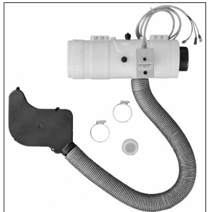
Abb. 10: Kompakt-Anschluss Set DN80/125 für raumlufunabhängigen Betrieb des Blaubrenners BNR 100.
