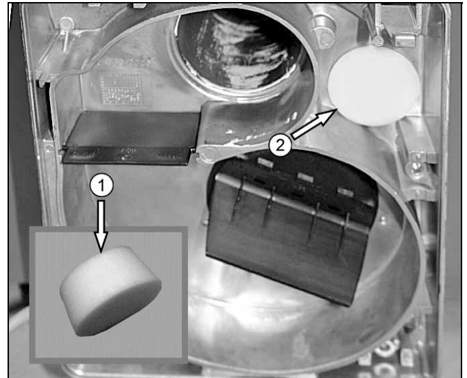
Abb. 19: Silikonstopfen lose und eingesteckt
