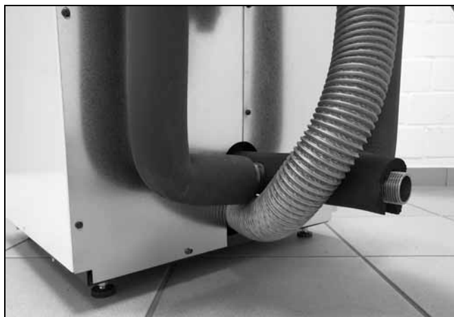
Abb. 14: Durchführung Zuluftschlauch
