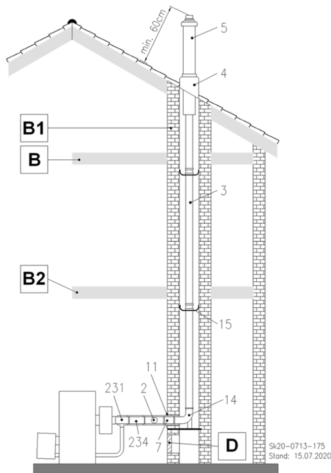
Abb. 53: C 93x Luft-Abgas-System im Schacht und Luft-Abgas-Rohrsystem mit Dachdurchführung
