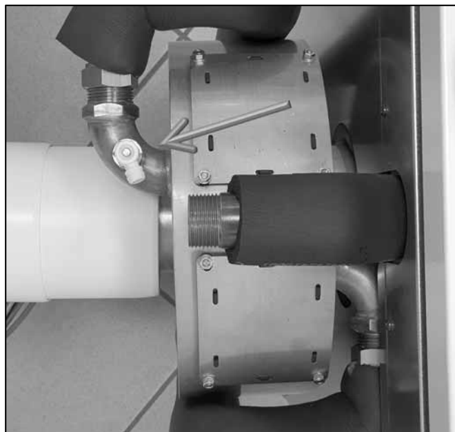
Abb. 24: Entlüfter am Abgaswärmetauscher
