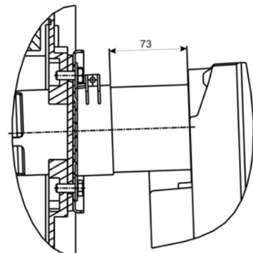
Abb. 20: Brennereinschubtiefe
