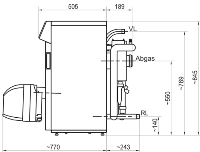
Abb. 2: Abmessungen
