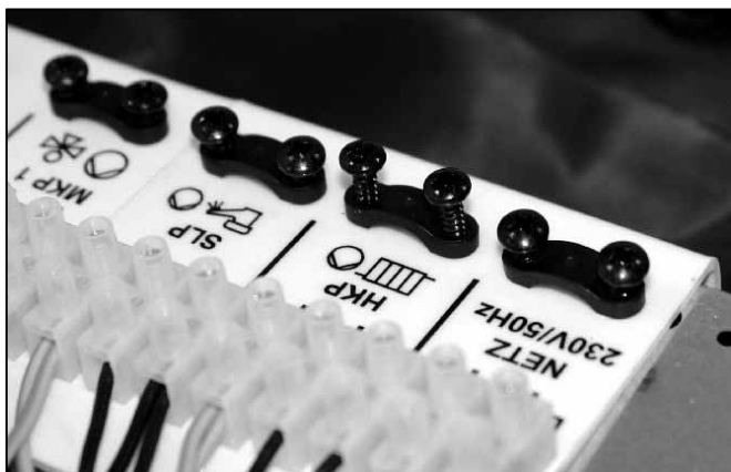
Abb. 25: Lüsterklemmen und Zugentlastungen
