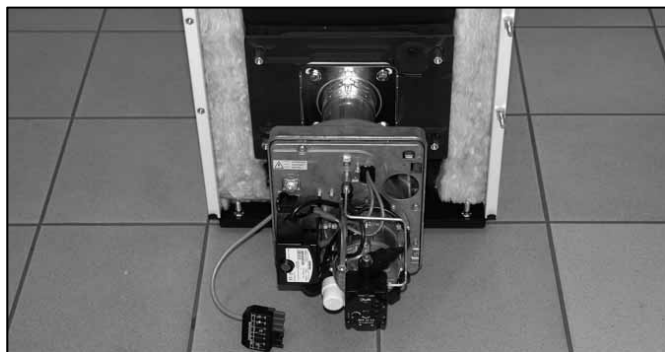
Abb. 22: Montierter Brenner BNR 100
