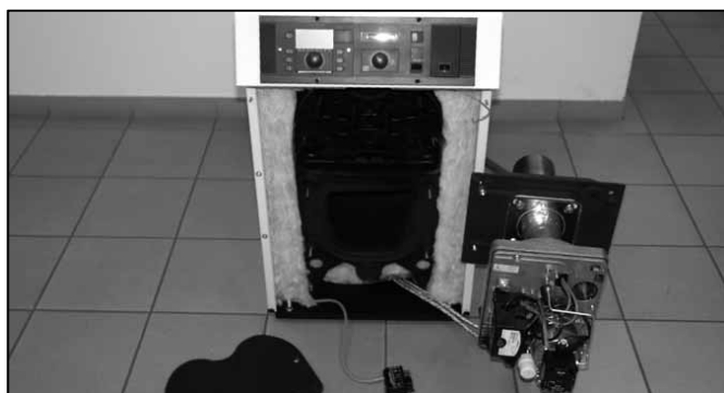
Abb. 83: Geöffneter Kessel mit Brenntür in Wartungsposition
