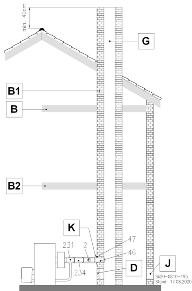
Abb. 46: B 33 Abgasrohr endet im feuchteunempfindlichen Schornstein
