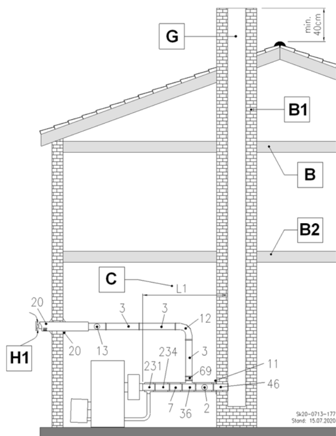
Abb. 52: C 83x Anschluss an einen feuchte-unempfindlichen Abgasschornstein und Zuluft durch die Außenwand
