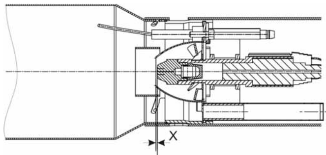
Abb. 77: "X"- Maß der Mischeinrichtung
