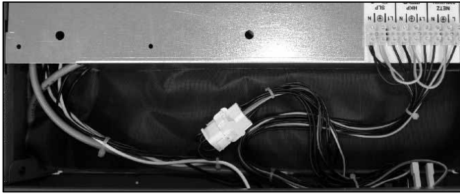
Abb. 29: Neunpoligen Brückenstecker öffnen. Das Gegenstück bleibt für die Notfunktion des Kessels im Schaltfeld.
