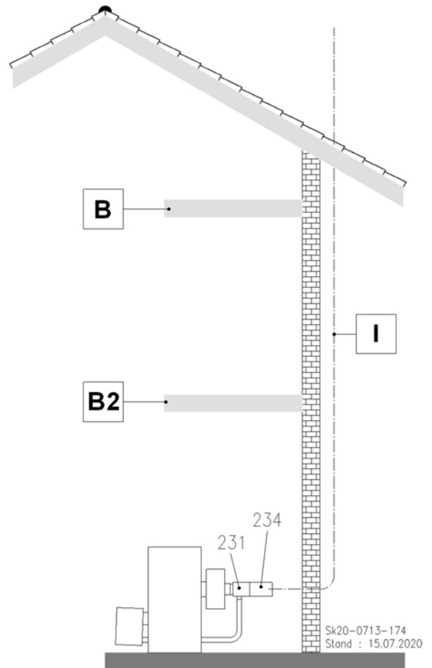
Abb. 51: C 63x Für Anschluss an eine nicht mit der Gasfeuerstätte geprüfte Verbrennungsluftzuführung und Abgasabführung
