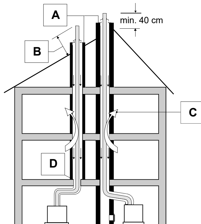
Abb. 43: Schachtqualität für Abgasleitungen
