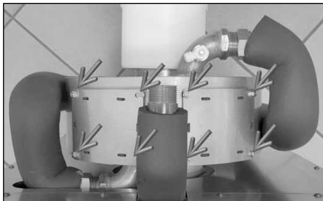
Abb. 81: Muttern der Reinigungsabdeckungen vom Abgaswärmetauscher
