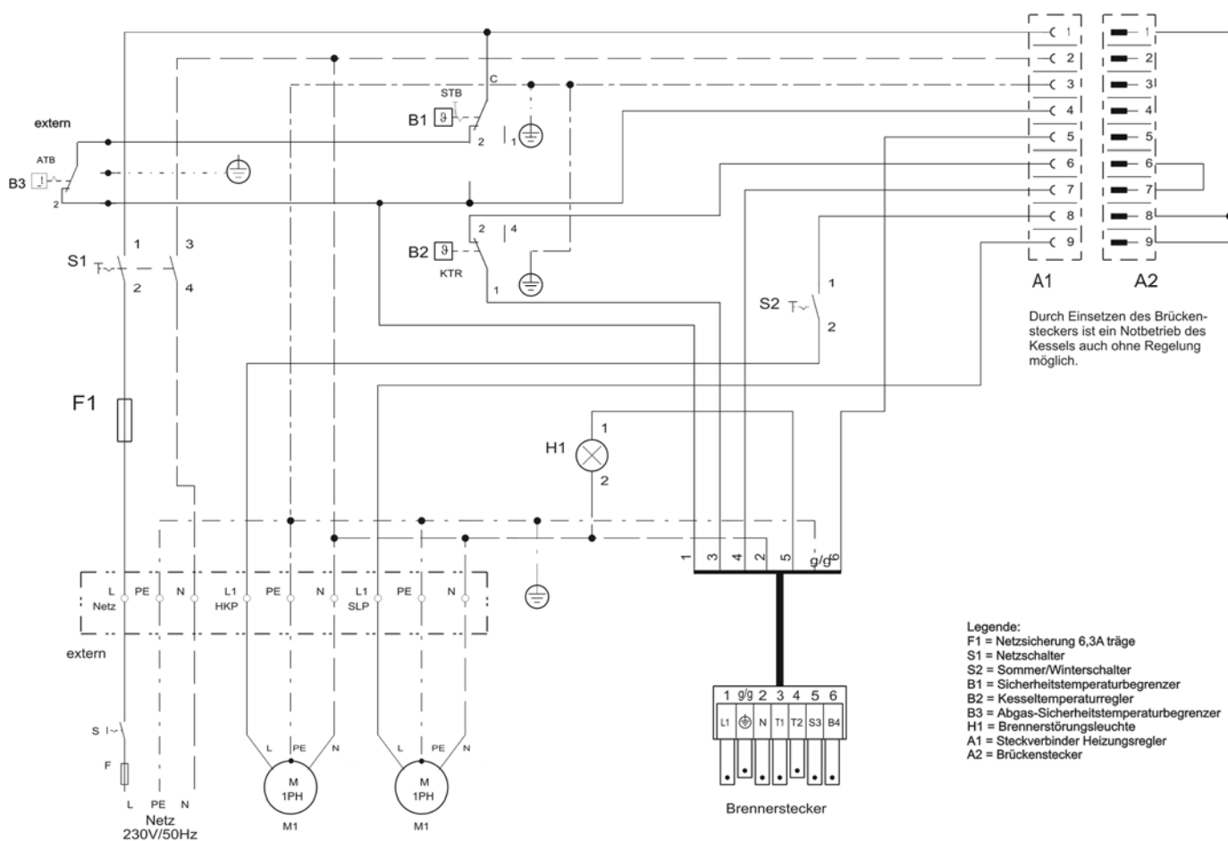
Abb. 39: Kessel-Grundschaftfeld ohne Regler: Elektrische Anschlüsse und Stromlaufplan
