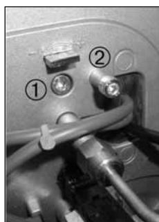
Abb. 74: Einstellung der Rezirkulation an der Stellschraube (1)
