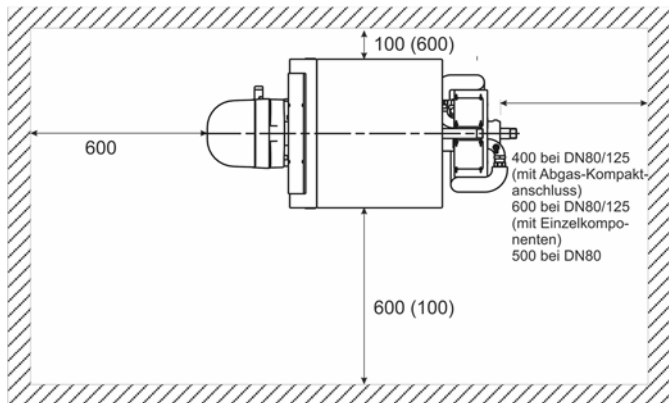
Abb. 1: Wandabstände bei horizontaler Abgasführung
