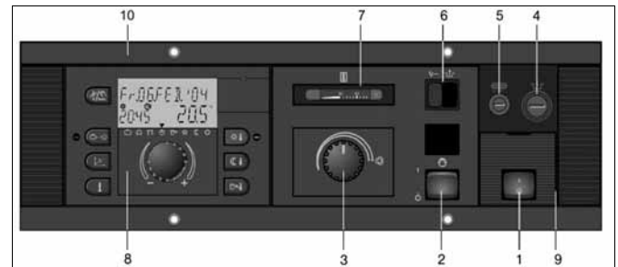
Abb. 71: Kesselgrundschaltfeld RATIOLINE PLUS
