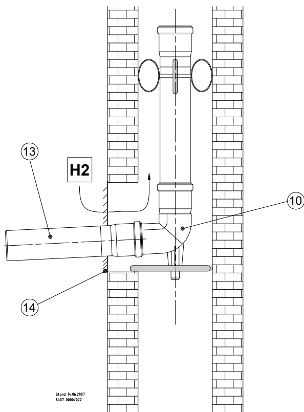
Abb. 60: Schachteinführung
