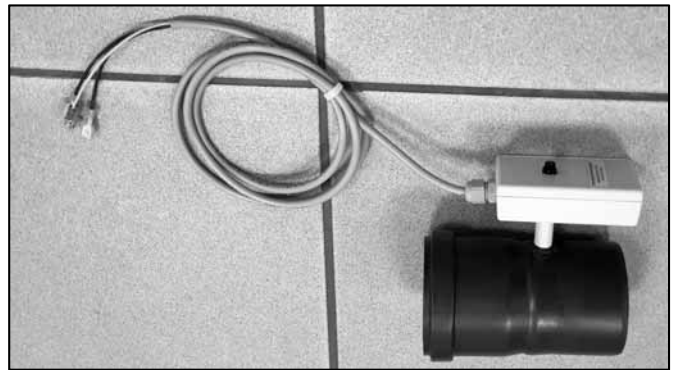
Abb. 33: Kesselanschluss DN80 mit Abgastemperaturbegrenzer
