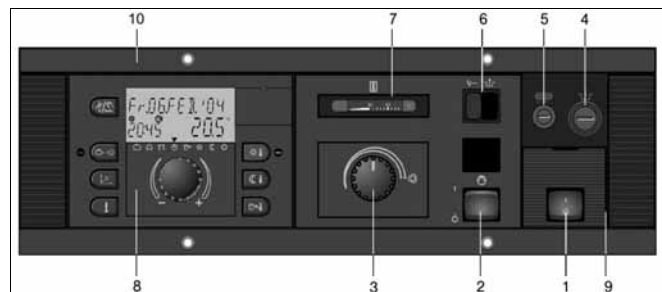
Abb. 71: Kesselgrundschaltfeld RATIOLINE PLUS
