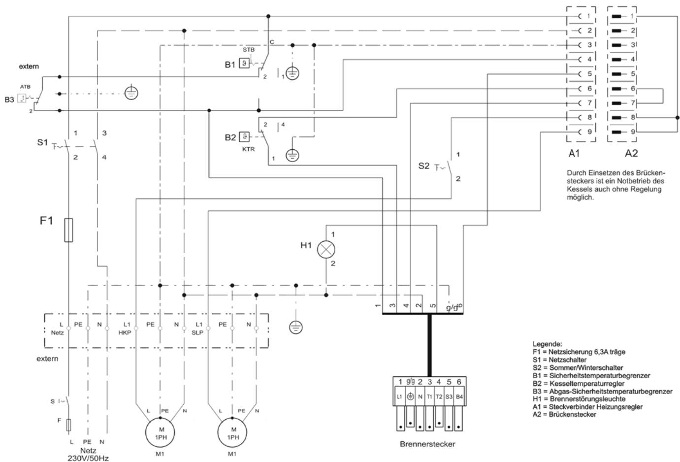
Abb. 39: Kessel-Grundschriftfeld ohne Regler: Elektrische Anschlüsse und Stromlaufplan
