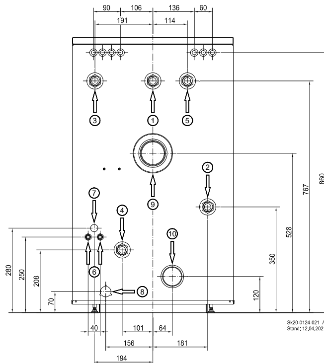
Abb. 3: Abmessungen Rückseite
