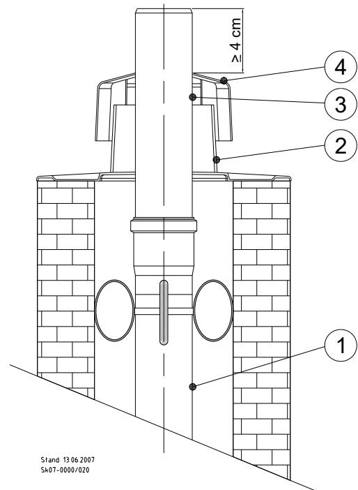
Abb. 58: Schachtabdeckung
