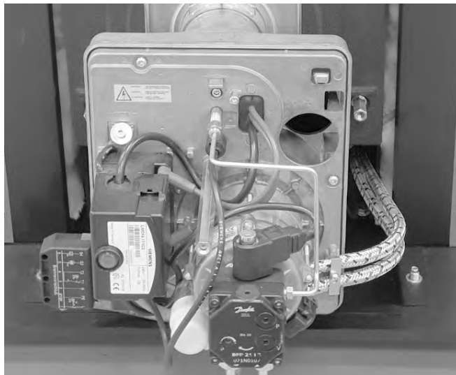
Abb. 94: Blaubrenner BNR 100 bzw. BNR 110
