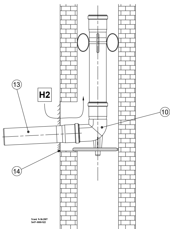
Abb. 59: Schachteinführung
