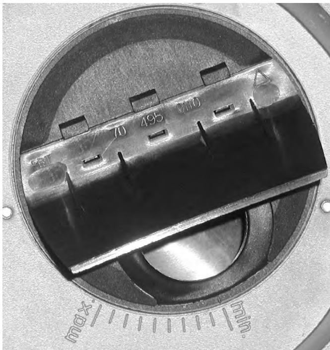
Abb. 74: Lufteinlaufdüse
