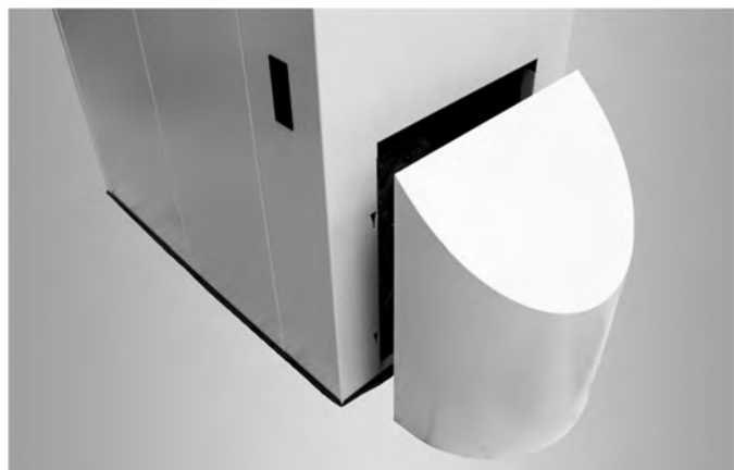
Abb. 81: Demontage der Brennerhaube
