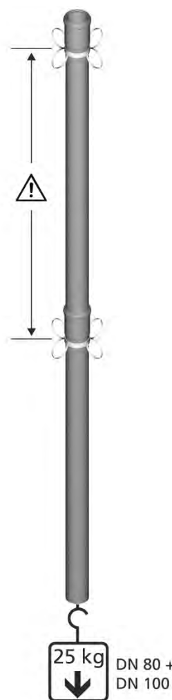
Abb. 56: Abgasrohre mit Stopping-Technik ①
