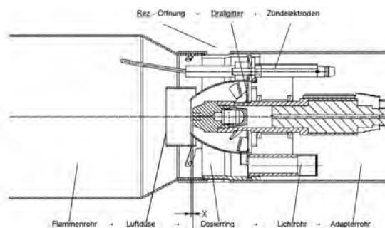
Abb. 95: Die Elektroden sind ca. 10 mm nach oben gebogen.
