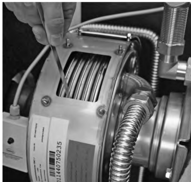
Abb. 91: Anwendung der Reinigungsklinge
