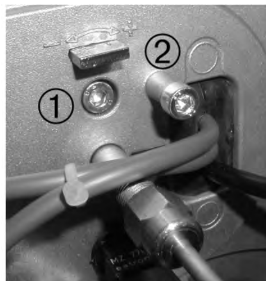
Abb. 73: Einstellschraube für die Rezirkulation (1)
