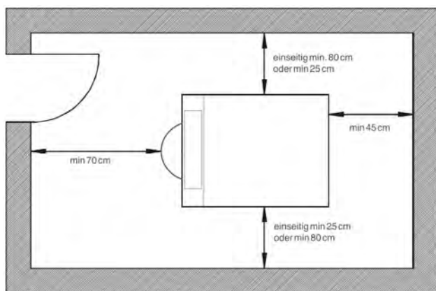
Abb. 1: Empfohlene Wandabstände
