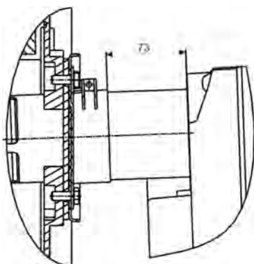
Abb. 71: Brenner-Einschubtiefe
