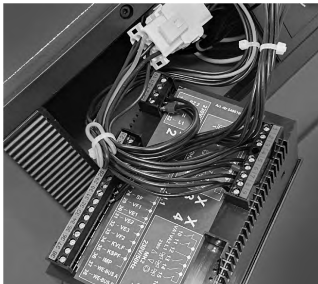
Abb. 35: Gesteckte Anschlussstecker.
