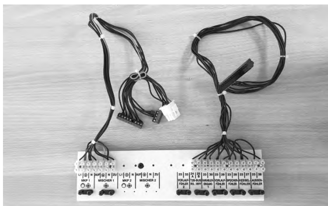
Abb. 31: Regler-Kabelbaum mit Klemmen und Steckverbinder zum Kesselschufeld.
