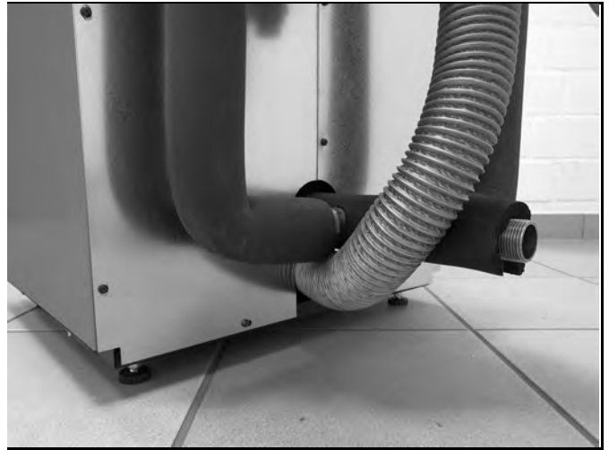
Abb. 14: Durchführung Zuluftschauch
