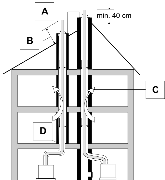
Abb. 43: Schachtqualität für Abgasleitungen
