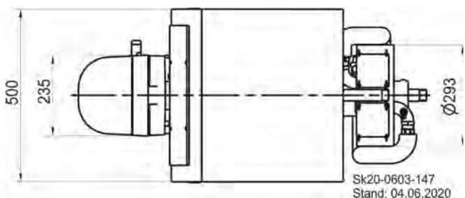
Abb. 3: Abmessungen
