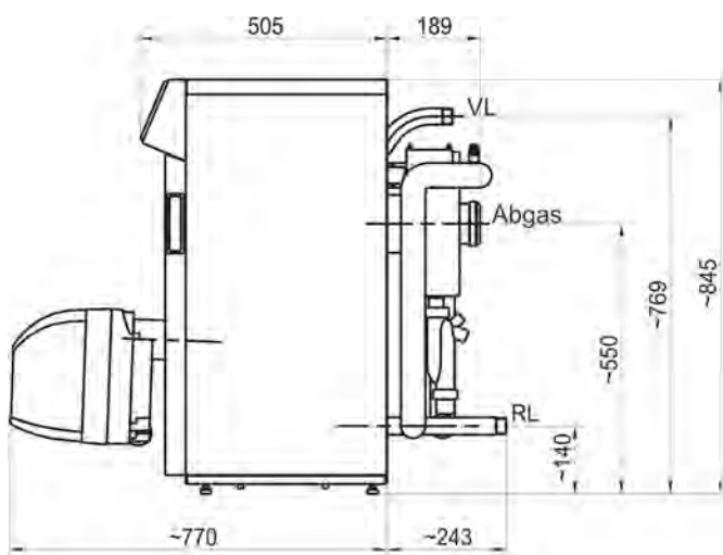
Abb. 2: Abmessungen
