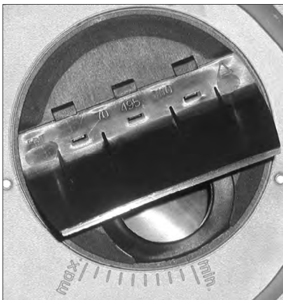
Abb. 75: Lufterlaufdüse
