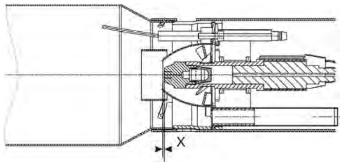
Abb. 77: "X"- Maß der Mischeinrichtung
