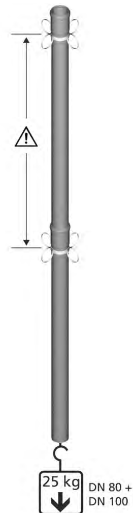
Abb. 57: Abgasrohre mit Stopping
