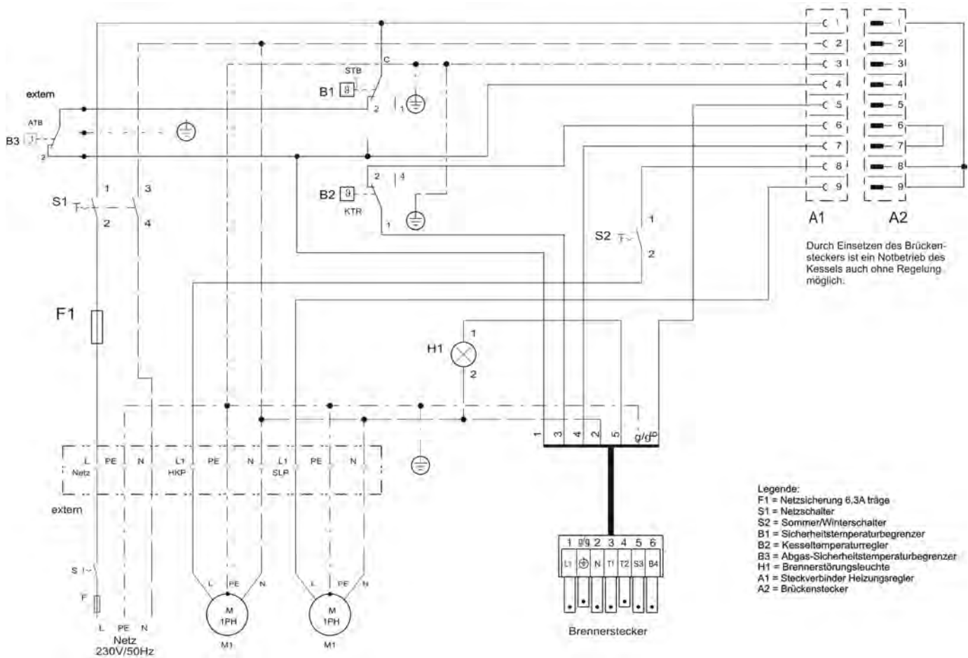
Abb. 39: Kessel-Grundschaltfeld ohne Regler: Elektrische Anschlüsse und Stromlaufplan
