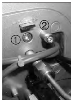
Abb. 74: Einstellung der Rezirkulation an der Stellschraube (1)
