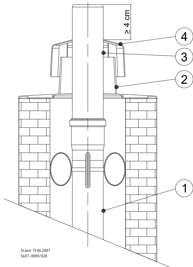
Abb. 59: Schachtabdeckung
