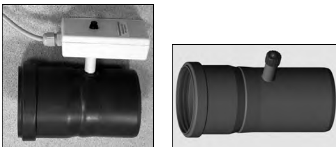
Abb. 9: Kesselanschluss-Set DN80 mit Messelement
