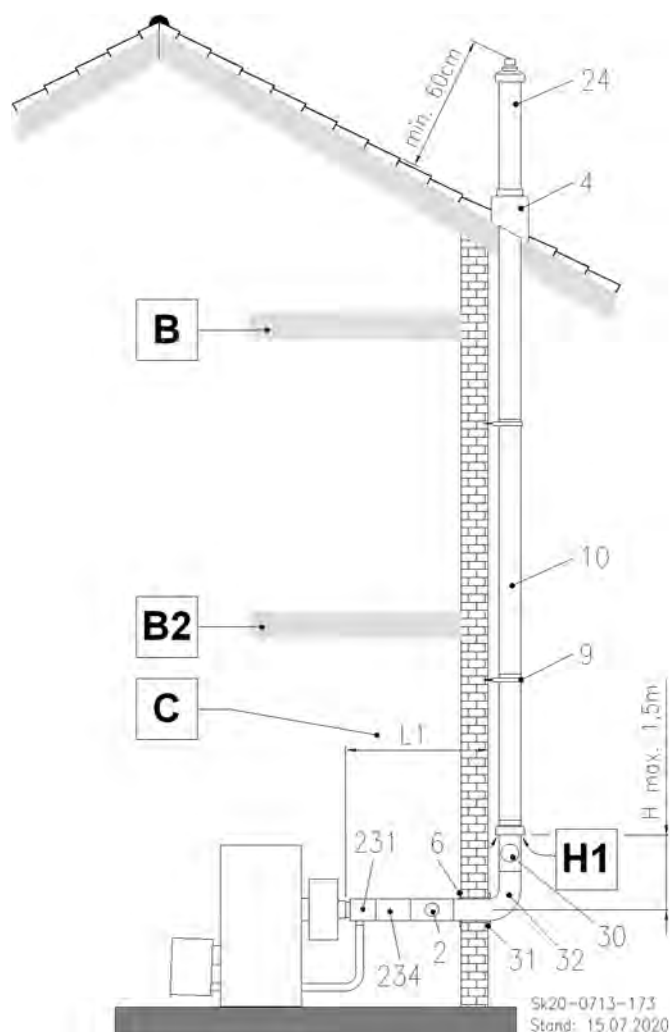
Abb. 50: C 53x Außenwandführung LAS
