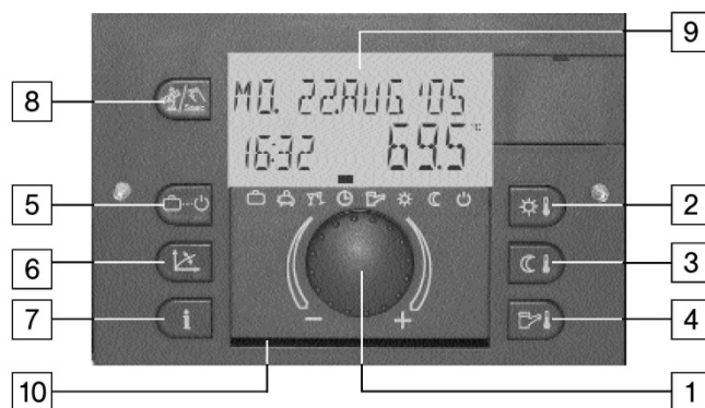
Abb. 5: Bedieneinheit
