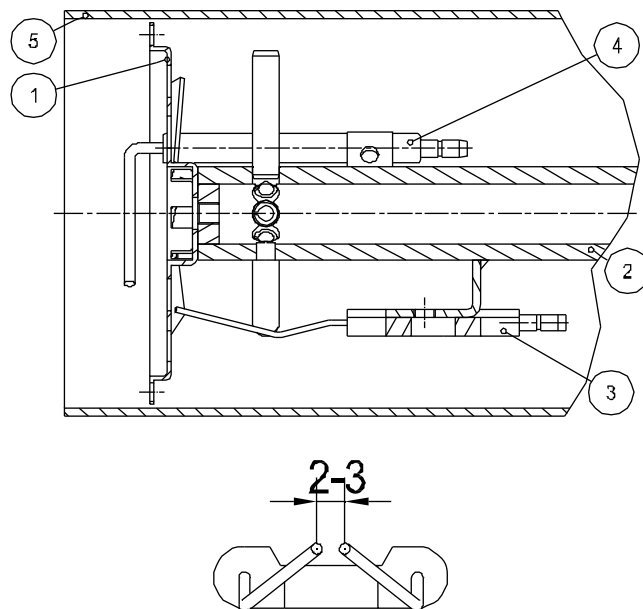
Abb. 17: Zündelectrodenpositionierung
