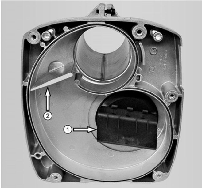
Abb. 9: Lufteinlaufdüse (1) mit Winkel und Luftklappe (2)
