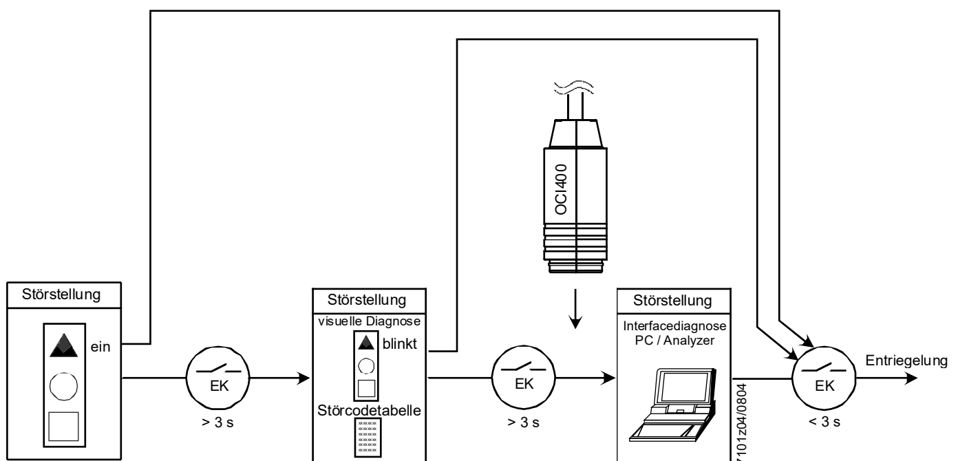
Abb. 25: Aktivierung der Störsachendiagnose (EK = Entstörtaster)
