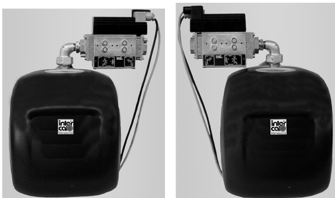
Abb. 4: Montierte Gasarmatur
