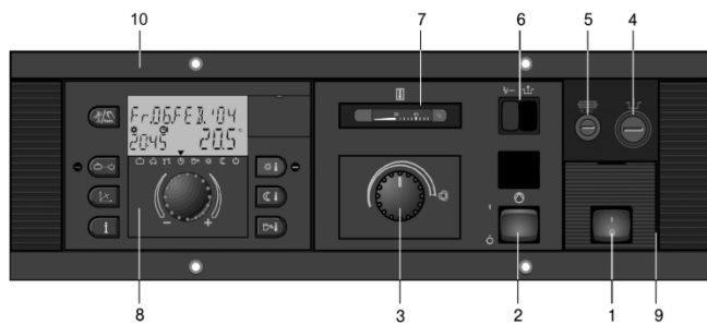
Abb. 1: Kesselgrundschaltfeld ECOHEAT Plus
