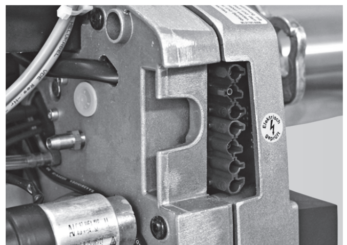
Abb. 5: Euro-Anschluss-Stecker
