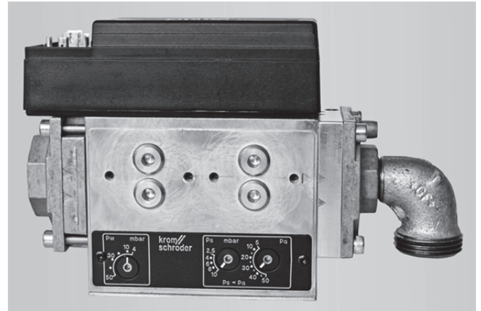
Abb. 11: Gasarmatur
