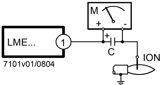
Abb. 22: Mess-Schaltung
