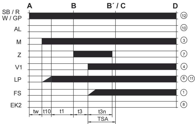
Abb. 13: Programmablauf LME 11.330
