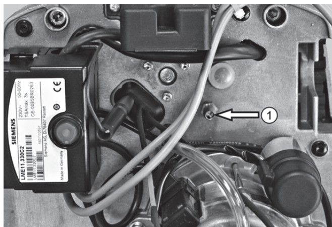
Abb. 8: Messnippel (Messing) zur Bestimmung der Gebläsepression
