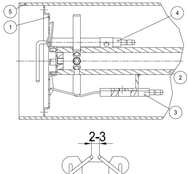
Abb. 17: Zündeletrodenpositionierung
