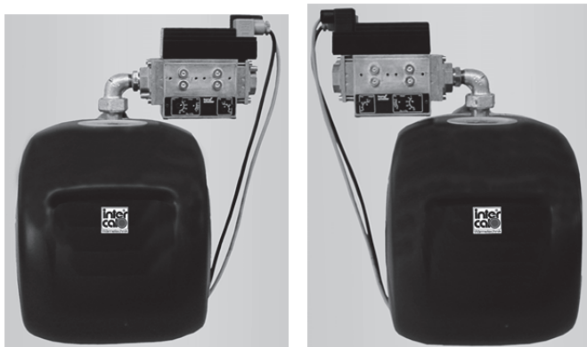
Abb. 4: Montierte Gasarmatur
