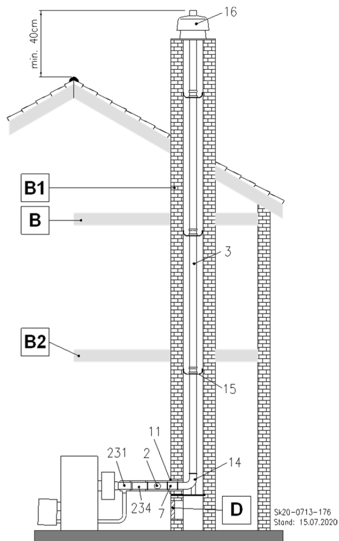
Abb. 56: C 93x Abgasrohr im Schacht
