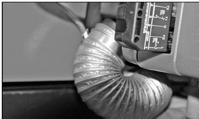
Abb. 23: Montage des RLU-Zuluftschlauchs
