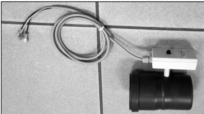
Abb. 35: Kesselanschluss DN 80 mit Abgastemperaturbegrenzer
