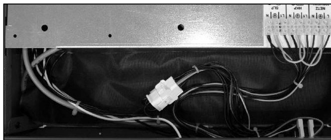
Abb. 31: Neunpoligen Brückenstecker öffnen. Das Gegenstück bleibt für die Notfunktion des Kessels im Schaltfeld.
