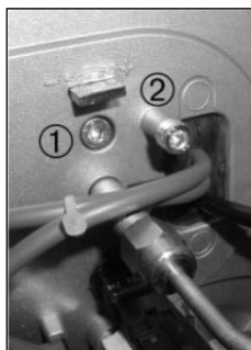
Abb. 76: Einstellung der Rezirkulation an der Stellschraube (1)
