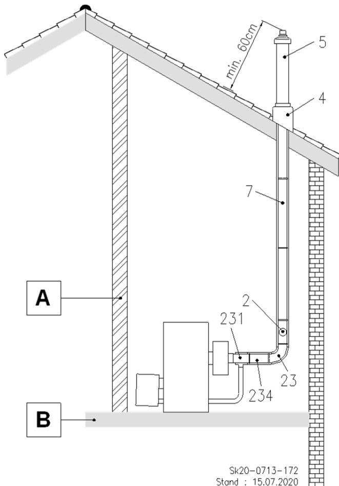
Abb. 51: C 33x Dachheizzentrale mit der Durchführung senkrecht durch ein Schrägdach
