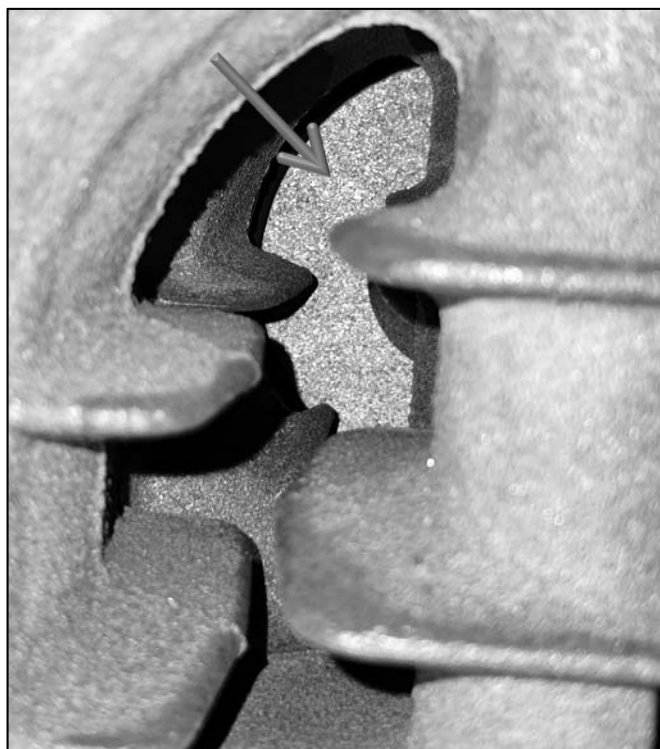
Abb. 86: Schalldämpfer im mittleren Zug
