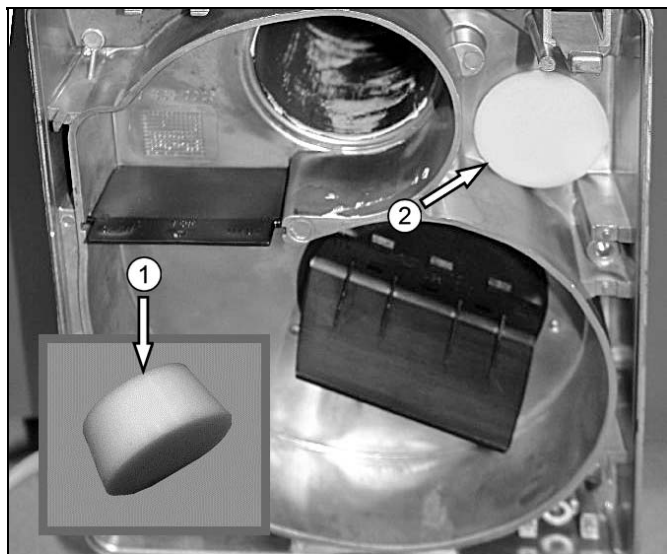
Abb. 21: Silikonstopfen lose und eingesteckt
