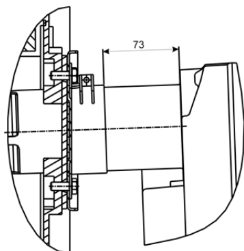
Abb. 74: Brenner-Einschubtiefe
