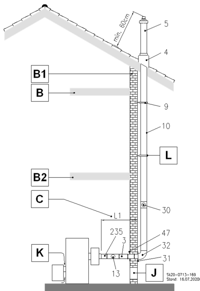
Abb. 46: B 23 Abgasrohr an der Außenwand
