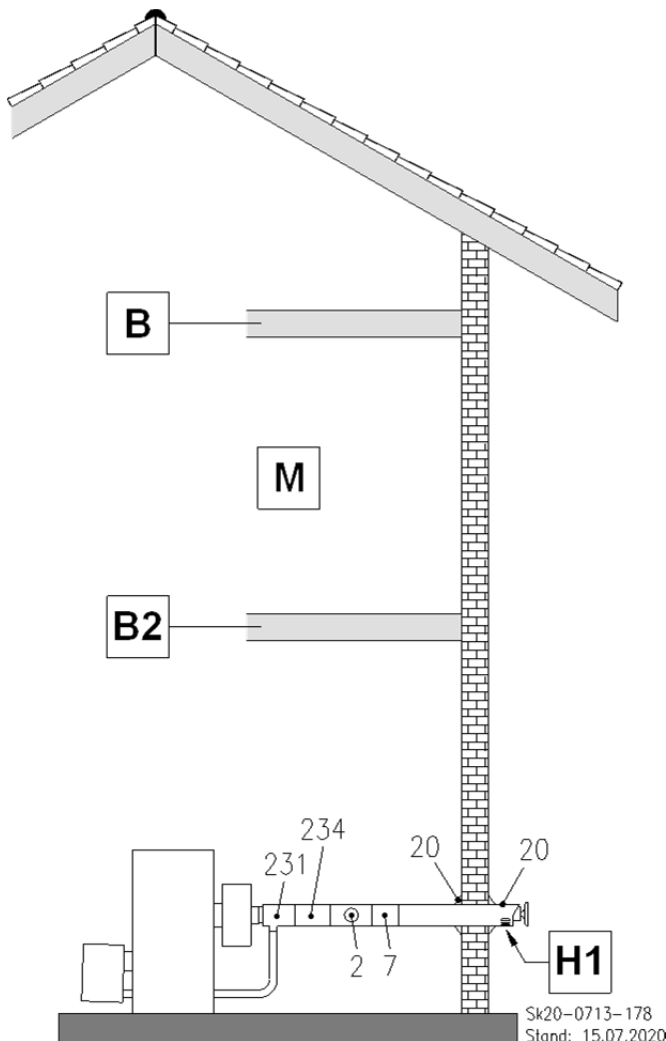
Abb. 49: C 13x Luft-Abgas-Rohrsystem horizontal durch die Außenwand
