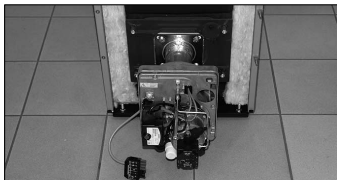
Abb. 24: Montierter Brenner BNR 100
