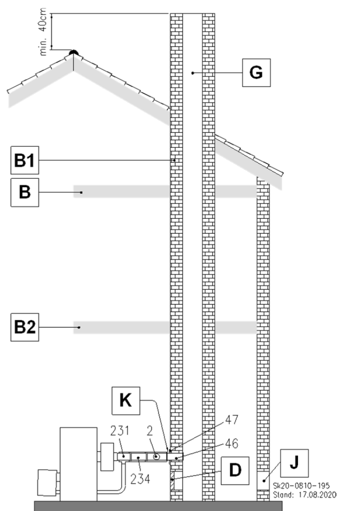
Abb. 48: B 33 Abgasrohr endet im feuchteunempfindlichen Schornstein
