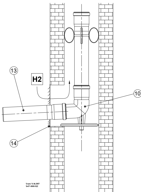
Abb. 62: Schachteinführung
