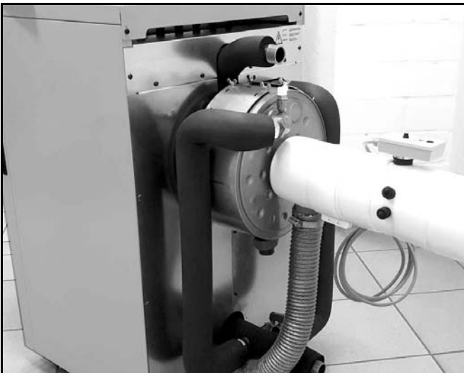
Abb. 17: Montierter Kesselanschluss DN 80/125 inkl. Abgastemperaturbegrenzer
