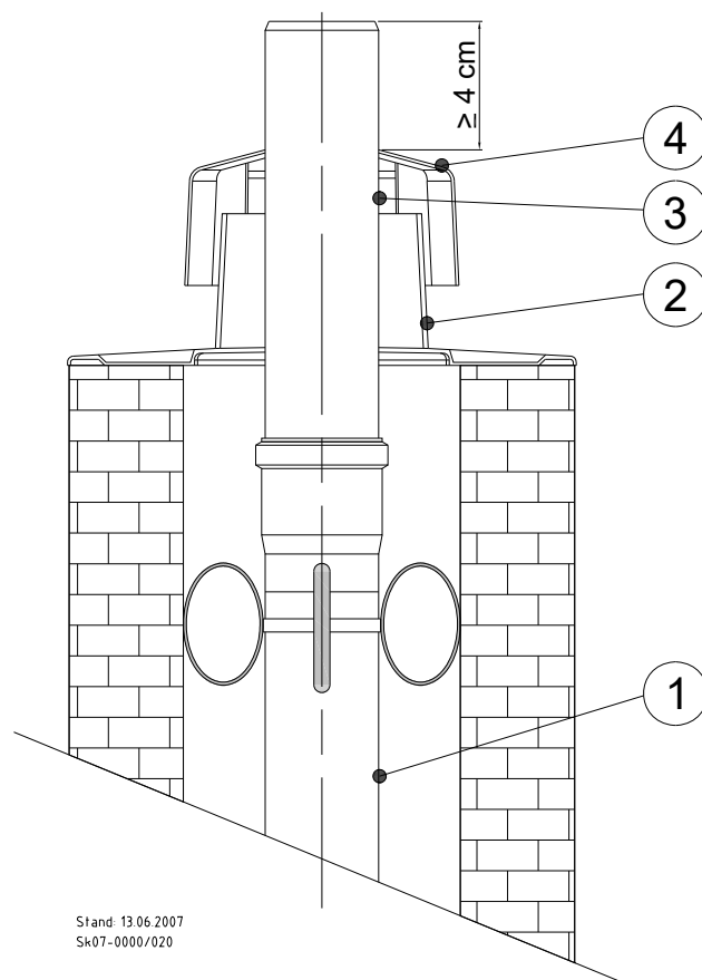
Abb. 61: Schachtabdeckung
