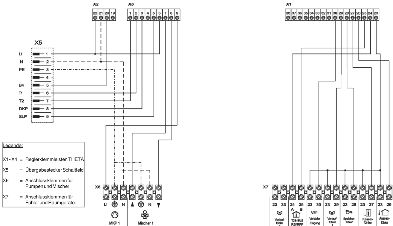
Abb. 42: Schaltplan Regleranschlusskabelbaum für THETA+ 2B und THETA+ 23B
