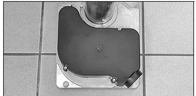
Abb. 19: Am Brenner vorhandener Schalldämpfer ohne Luftstutzen
