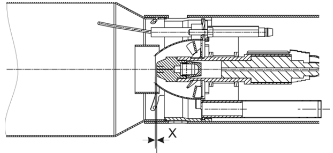
Abb. 79: "X"- Maß der Mischeinrichtung
