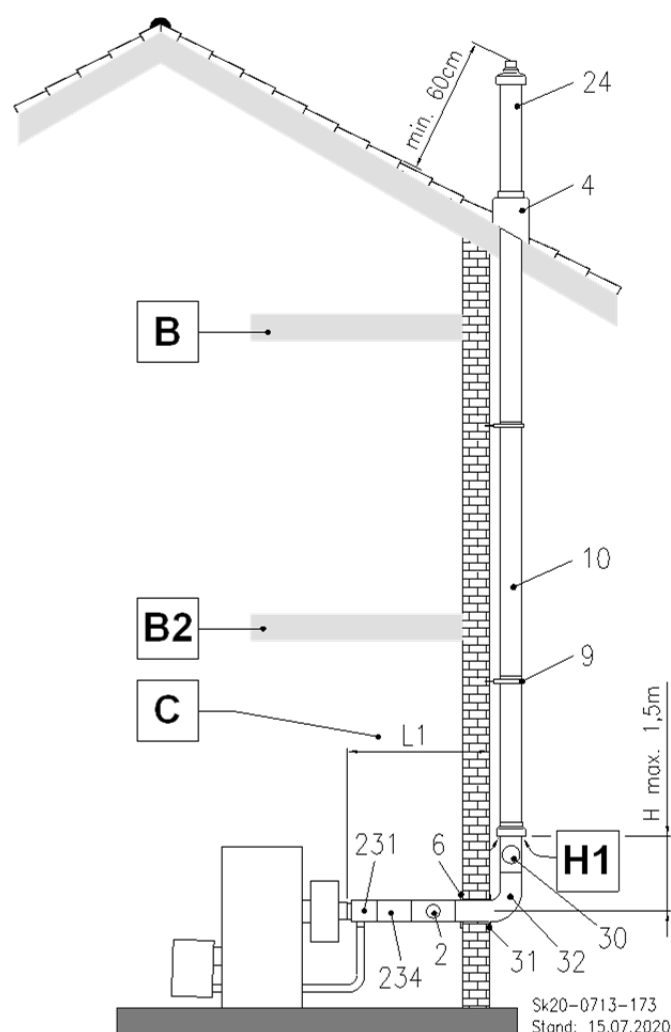
Abb. 52: C 53x Außenwandführung LAS
