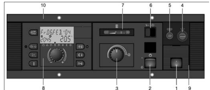
Abb. 73: Kesselgrundschaltfeld RATIOLINE PLUS
