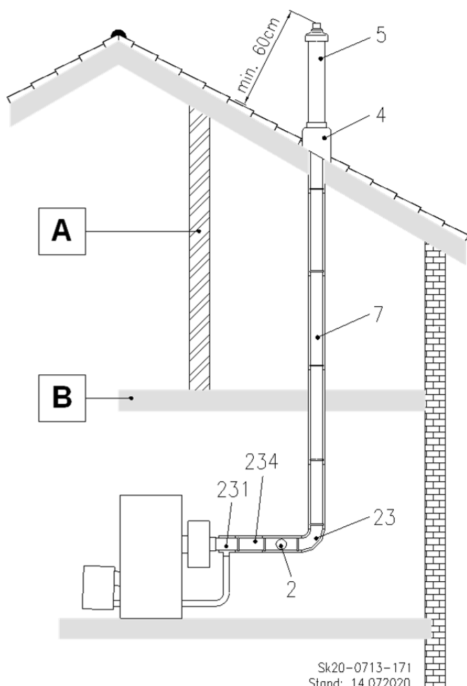
Abb. 50: C 33x Luft-Abgas-Rohrsystem senkrecht durch eine Decke und eine Dachhaut
