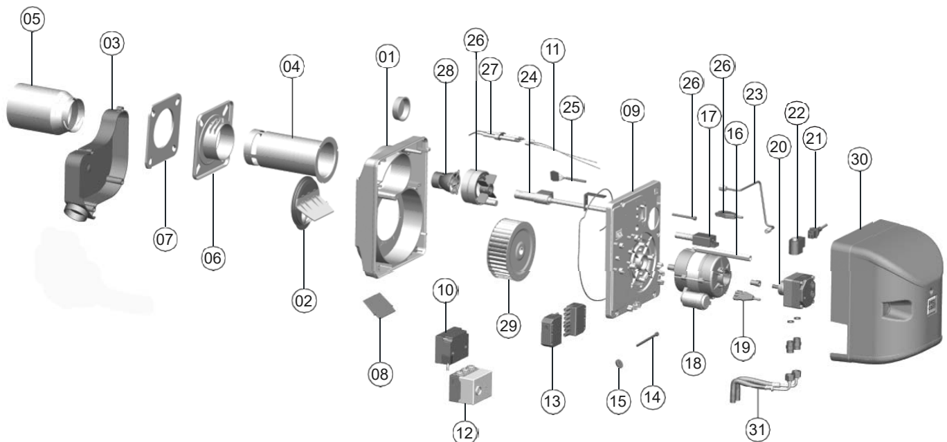
Abb. 97: Explosionsdarstellung Ölbrenner BNR 100
