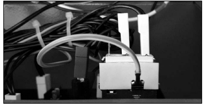
Abb. 38: Aufsicht Kessel-Sicherheitstemperaturbegrenzer (STB) (rechts oben im Kesselschaltfeld)
