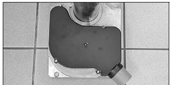
Abb. 20: Am Brenner montierter Schalldämpfer mit Luftstutzen
