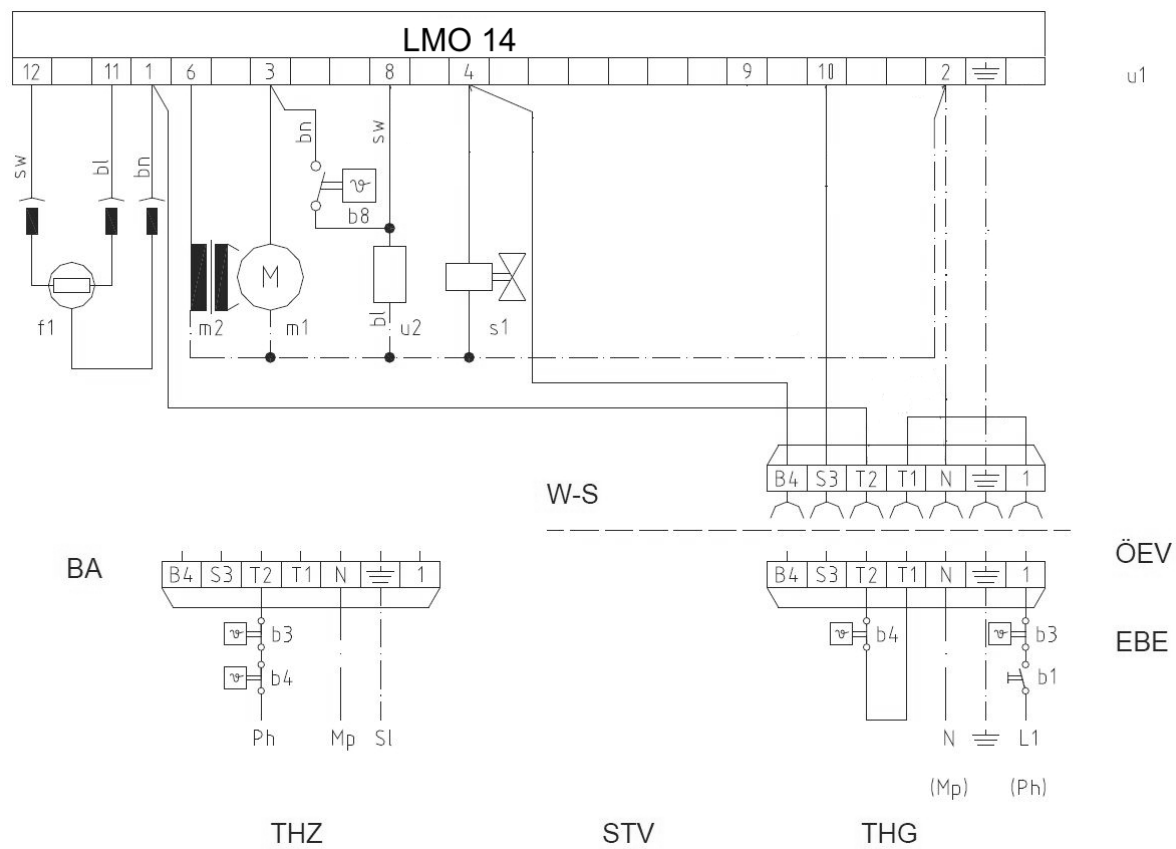
Abb. 44: Schaltplan Blaubrenner BNR 100 mit Siemens Feuerungsautomat LMO 14
