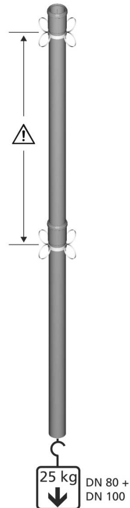
Abb. 59: Abgasrohre mit Stoppring
