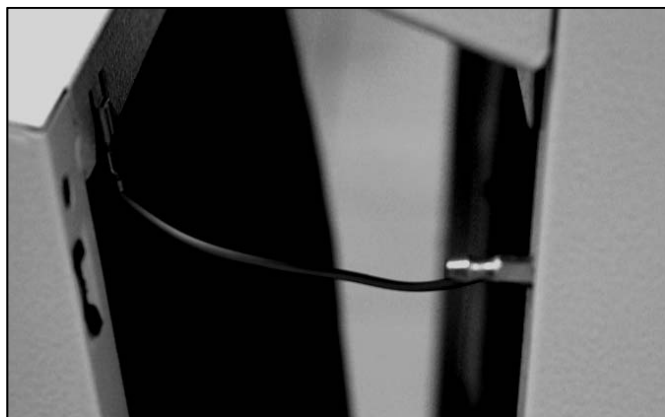
Abb. 28: Schutzleiter zwischen Frontverkleidung und Verkleidungsdeckel
