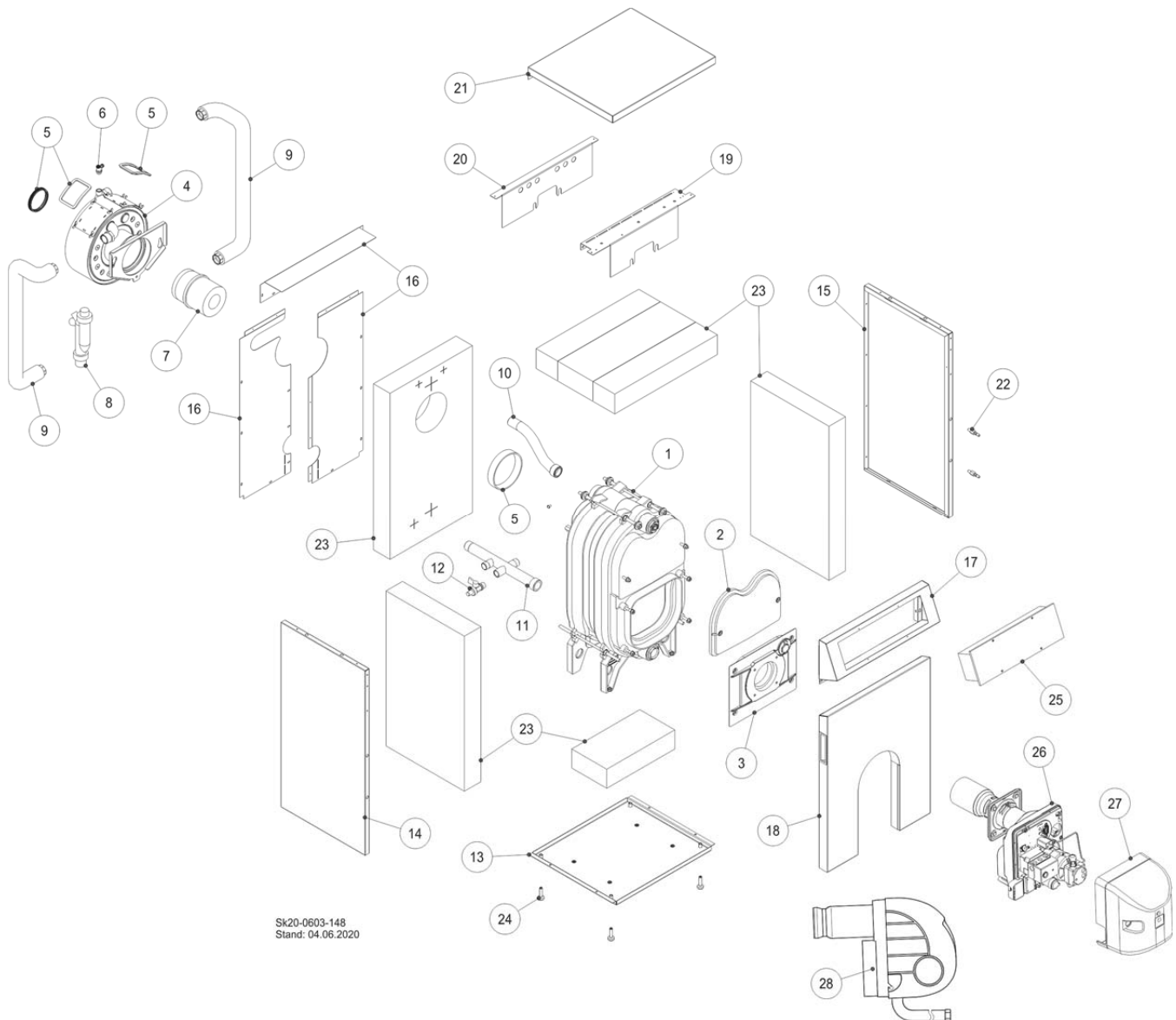
Abb. 96: Explosionsdarstellung RATIOLINE Plus
