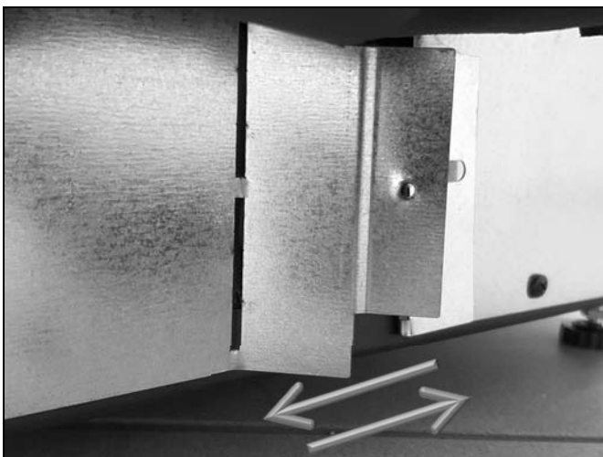
Abb. 13: Herausbrechen des vorgestanzten Ausschnitts
