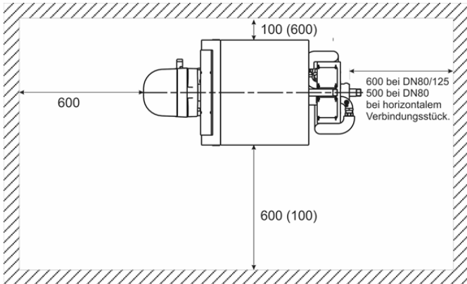
Abb. 1: Wandabstände
