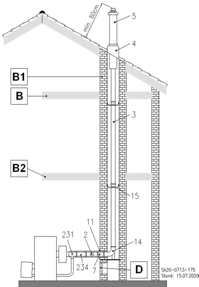
Abb. 55: C 93x Luft-Abgas-System im Schacht und Luft-Abgas-Rohrsystem mit Dachdurchführung
