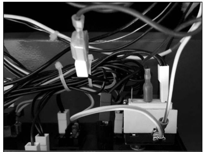
Abb. 40: Reihenschaltung der Sicherheitsthermostaten
