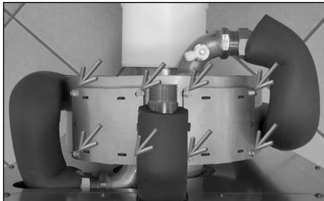
Abb. 83: Muttern der Reinigungsabdeckungen vom Abgaswärmetauscher
