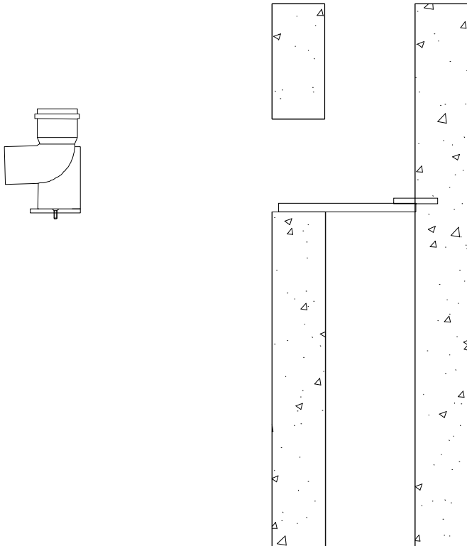
Abb. 58: 87° Stützbogen und Auflageschiene
