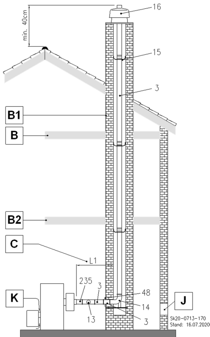
Abb. 47: B 23 Abgasrohr im Schornsteinschacht
