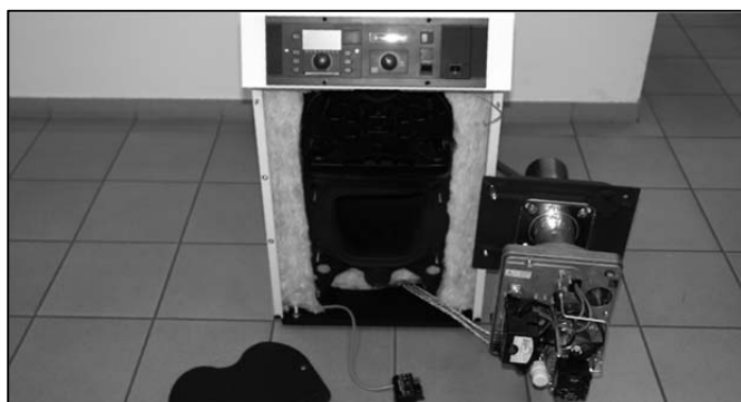
Abb. 85: Geöffneter Kessel mit Brenntür in Wartungsposition
