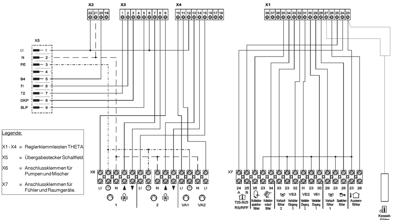
Abb. 43: Schaltplan Regleranschlusskabelbaum THETA+ 233B THETA+ 2233 BVVC-OT
