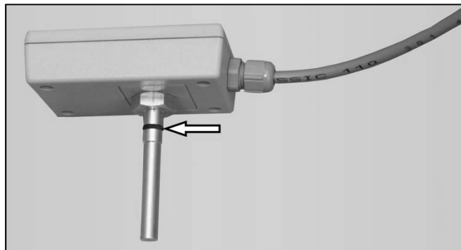
Abb. 92: Dichtung am Temperaturfühler des ATB DN 80
