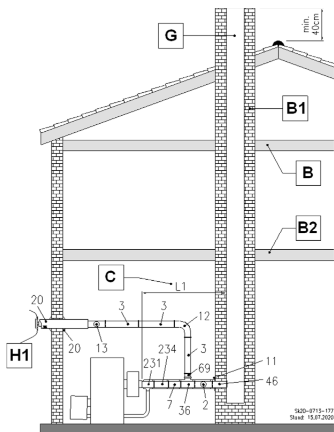
Abb. 54: C 83x Anschluss an einen feuchte-unempfindlichen Abgasschornstein und Zuluft durch die Außenwand
