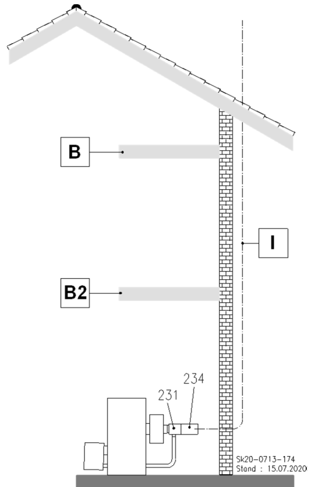
Abb. 53: C 63x Für Anschluss an eine nicht mit der Gasfeuerstätte geprüfte Verbrennungsluftzuführung und Abgasabführung
