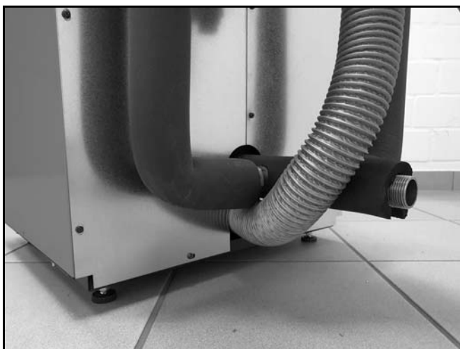
Abb. 15: Durchführung Zuluftschlauch
