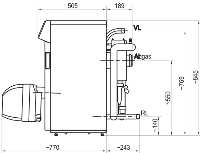
Abb. 2: Abmessungen
