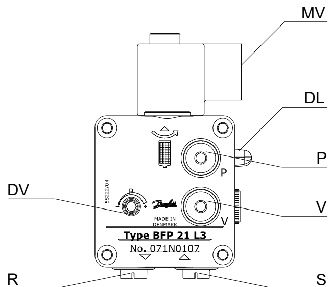
Abb. 80: Danfoss Ölpumpe BFP 21 L3 (Druckbereich 10-14 bar)
