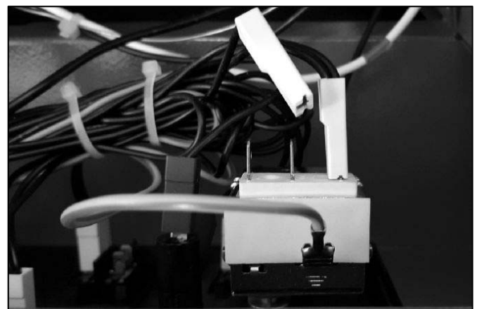
Abb. 39: Abgezogene mittlere Flachsteckhülse
