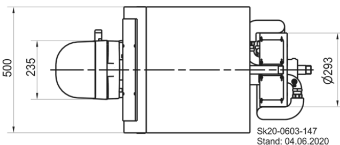
Abb. 3: Abmessungen
