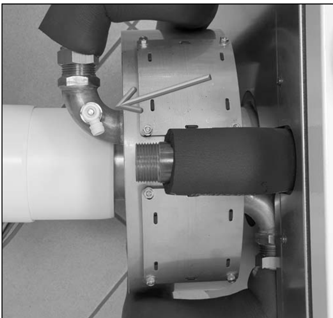
Abb. 26: Entlüfter am Abgaswärmetauscher
