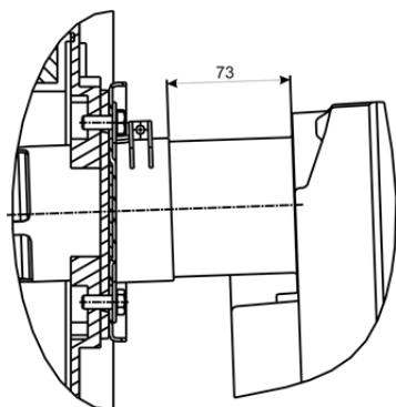
Abb. 22: Brennereinschubtiefe
