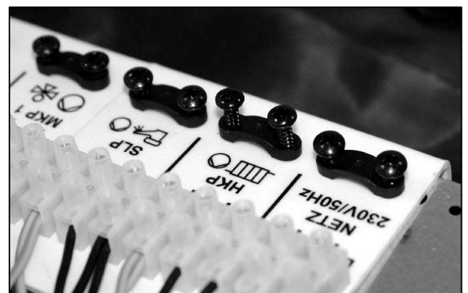
Abb. 27: Lüsterklemmen und Zugentlastungen
