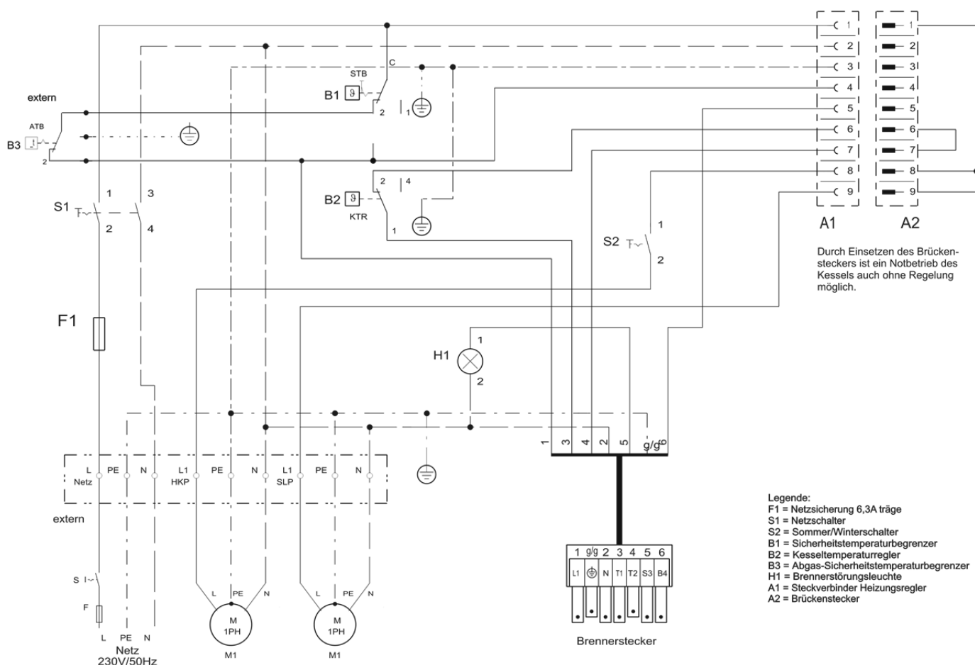
Abb. 41: Kessel-Grundschaftfeld ohne Regler: Elektrische Anschlüsse und Stromlaufplan
