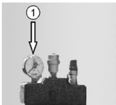
Abb. 3: Sicherheitsgruppe mit Manometer ①
